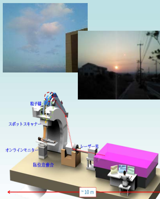
レーザー駆動の超小型粒子線がん治療装置のイメージ
