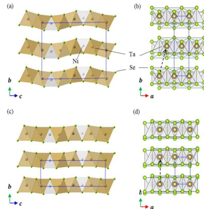
図1 (a)(b) 二方向から見た1気圧30℃における \text{Ta}_2\text{NiSe}_5 の結晶構造。(c)(d) 4万気圧-73℃における結晶構造。(b)(d)のb軸方向の上下の積層関係を見比べると、例えばTa原子の位置は(b)では斜め上にあるのに対して(d)では真上に位置しています(図中点線矢印)。これは層全体がスライドしたことに対応します。
