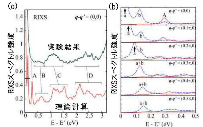
図2 RIXSスペクトル強度。a)実験結果と計算結果の比較。b)低エネルギーの計算結果。2種類の線(実線・破線)は異なる偏光の場合。
