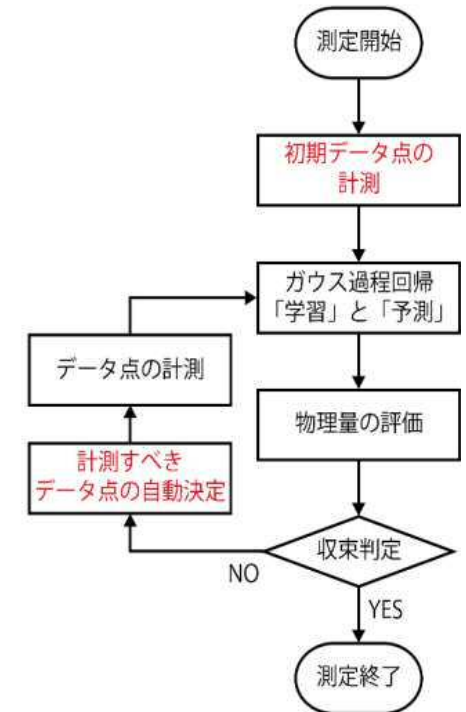
図1 従来型のX線スペクトル測定と今回開発した手法の比較。本手法では、ガウス過程回帰を用いて実験データを「学習」し、X線スペクトルを「予測」することで、計測すべきエネルギー点を自動的に決定することができます。
