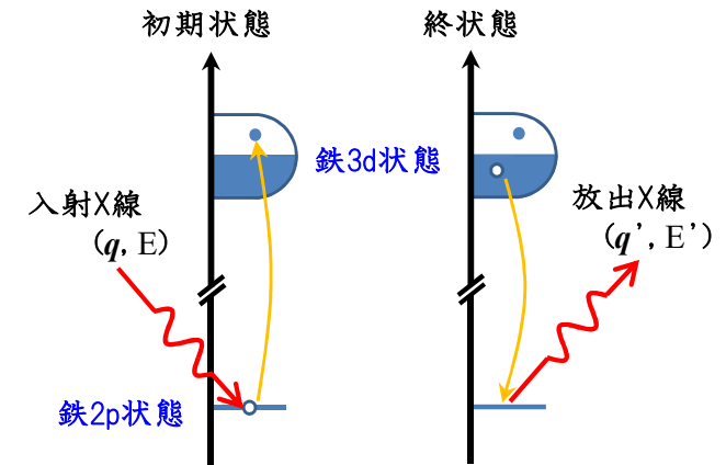
図1 共鳴非弾性X線散乱(RIXS)の模式図。
