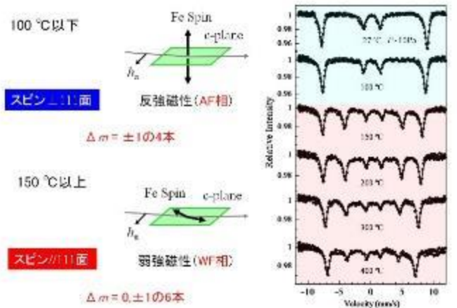
図2 イリジウムを0.1%添加した \alpha - \text{Fe}_2\text{O}_3 薄膜の斜入射放射光メスバウアー分光スペクトルの温度変化
