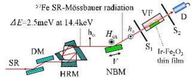
図1 ^{57}\text{Fe} -斜入射放射光メスバウアー分光の実験配置 放射光SRは二結晶分光器DM、高エネルギー分解能分光器HRM、鉄核分光器NBMを用いて15neVまで超高分解能化され、試料に斜入射する。全反射したX線がNaI検出器で検出され、吸収スペクトルが観測される。
