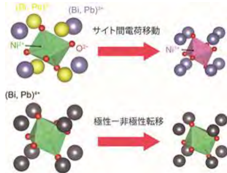
図： \text{Bi}_{1-x}\text{Pb}_x\text{NiO}_3 の負熱膨張メカニズム サイト間電荷移動と極性-非極性転移により 結晶が縮む様子を模式的に表しました。
