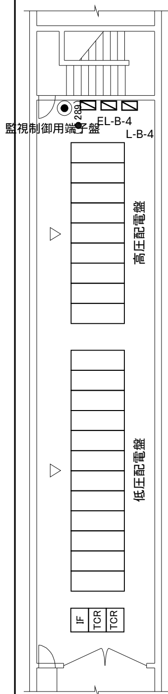
実験棟MB1F電気室Ⅱ平面略図
