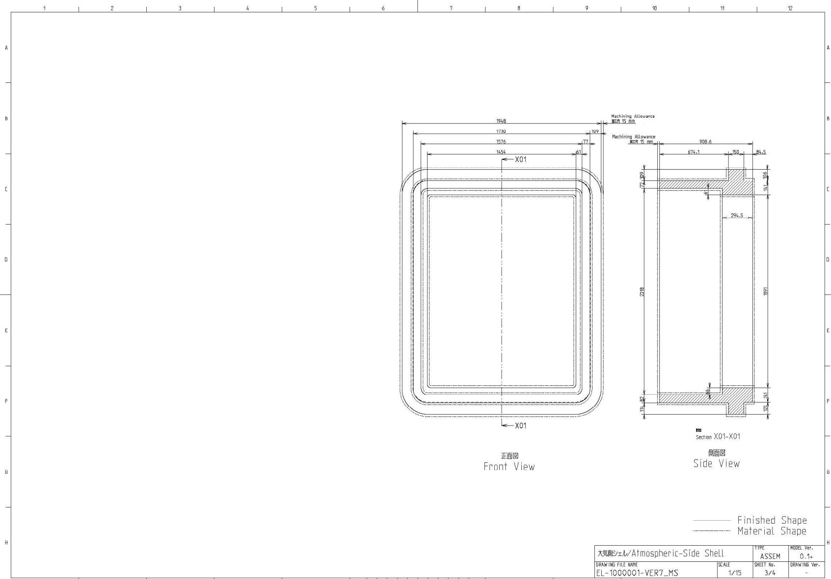
図2 余肉付き大気側シェル
