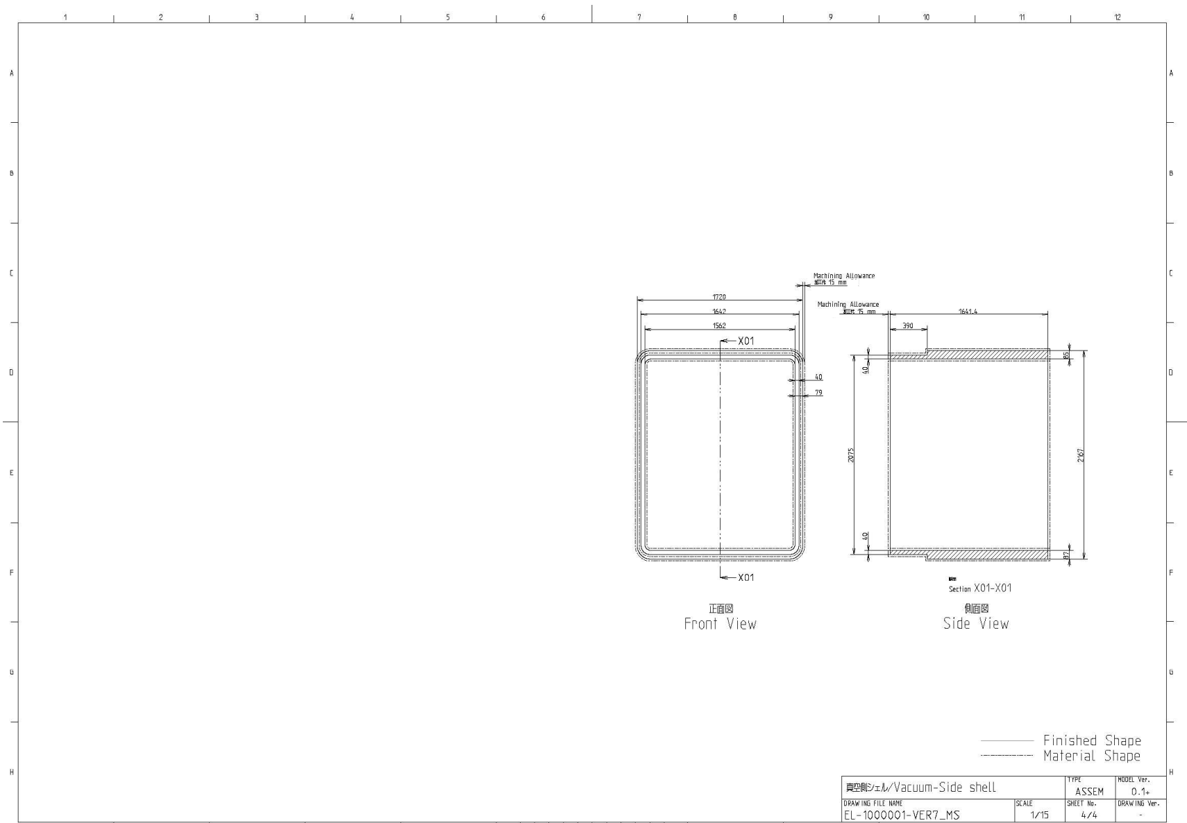
図3 余肉付き真空側シェル
