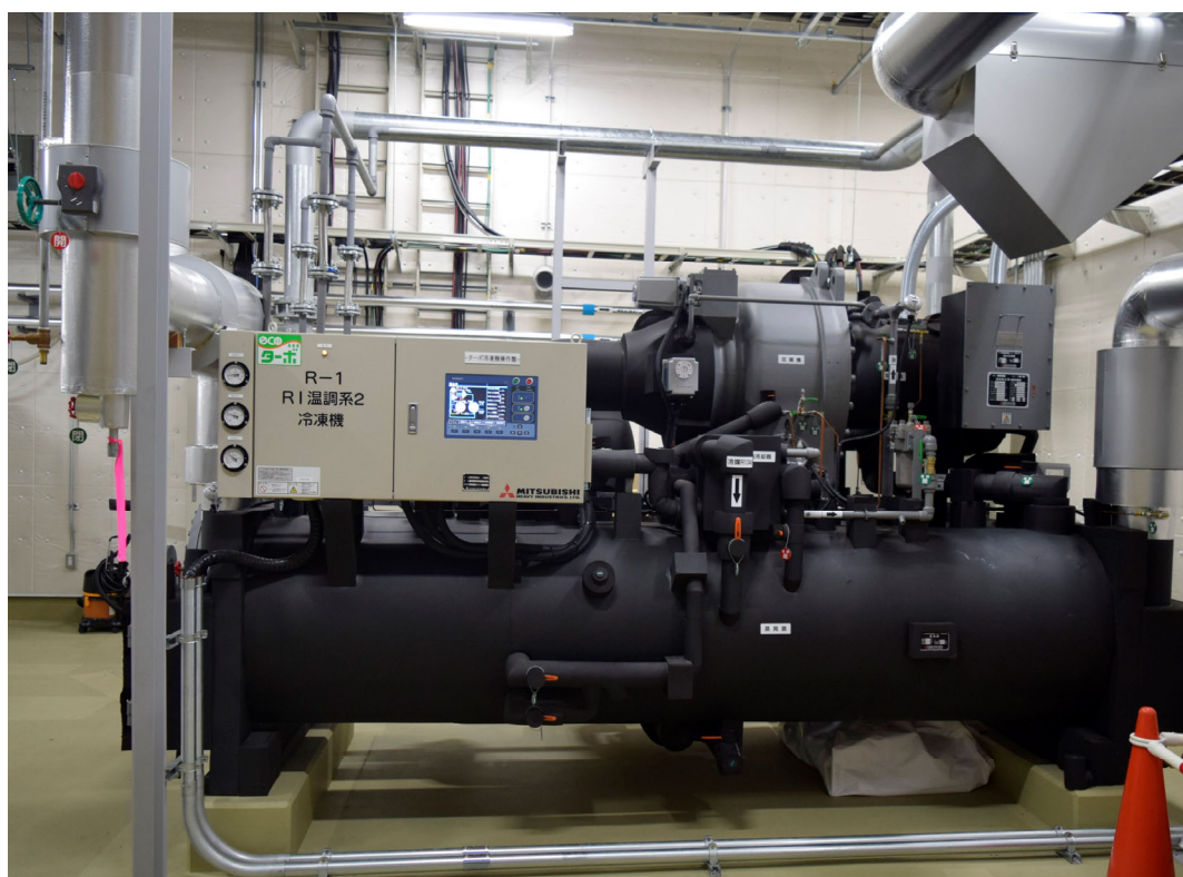
図1 作業対象設備外観
