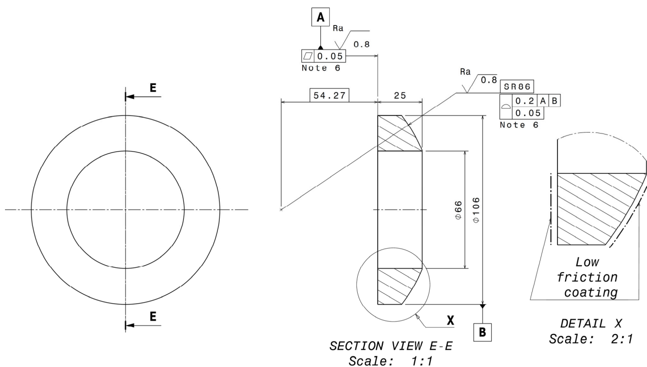
図 9 球面ワッシャ
