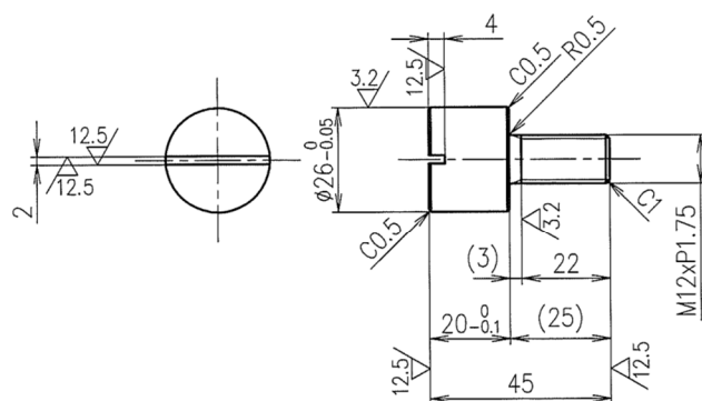
図 8 Spiralock 固定ピン
