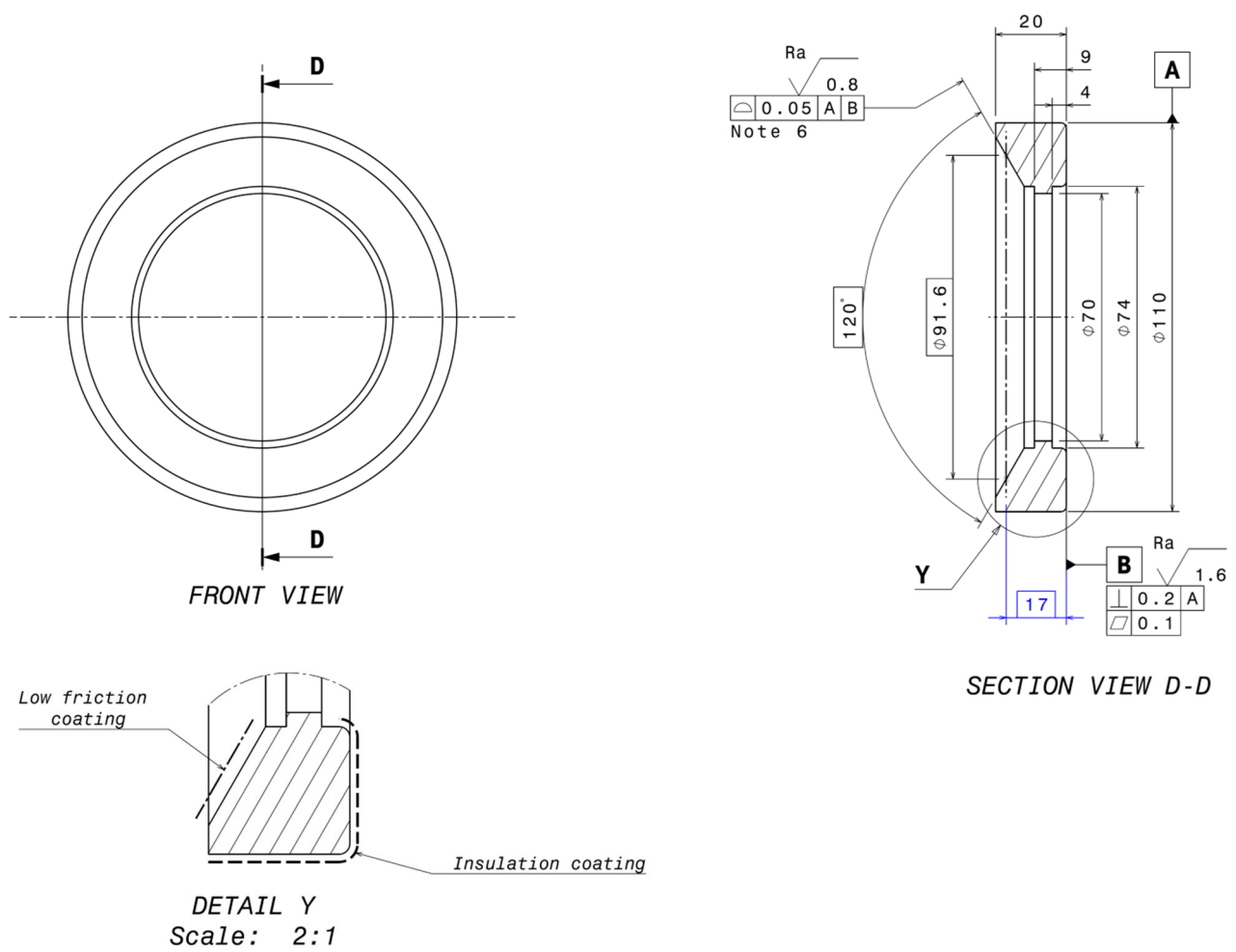
図 10 円錐ワッシャ
