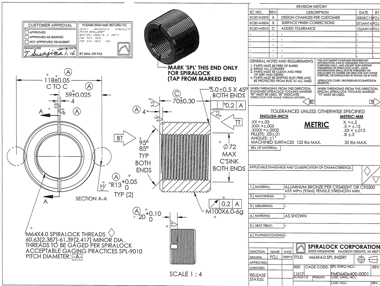
図 7 Spiralock インサート
