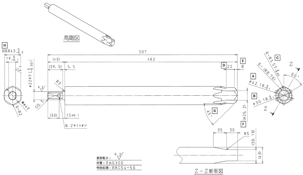
図 1 CB 締結用レンチ
