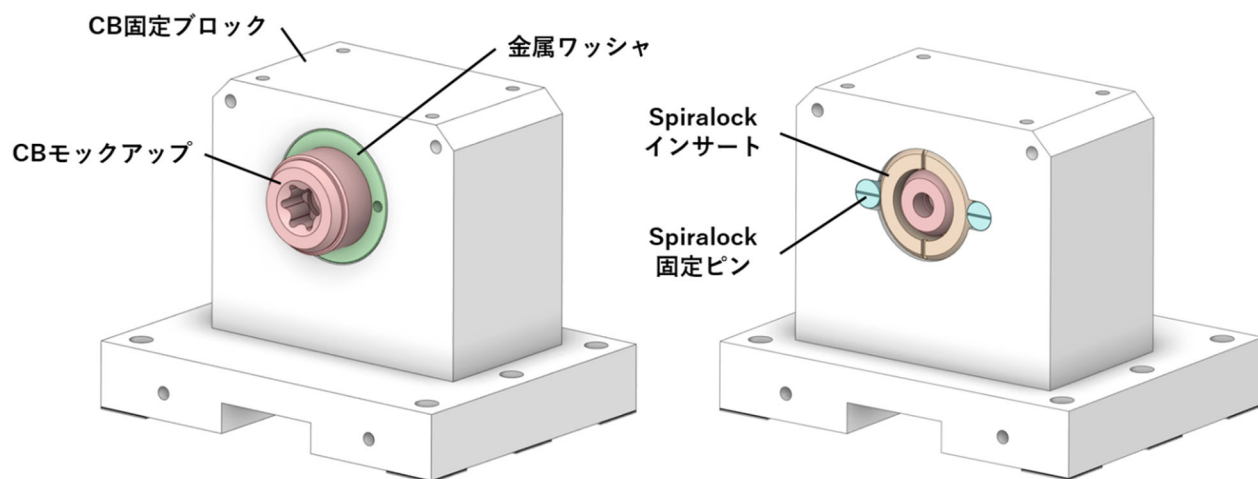
図 5 組立図
