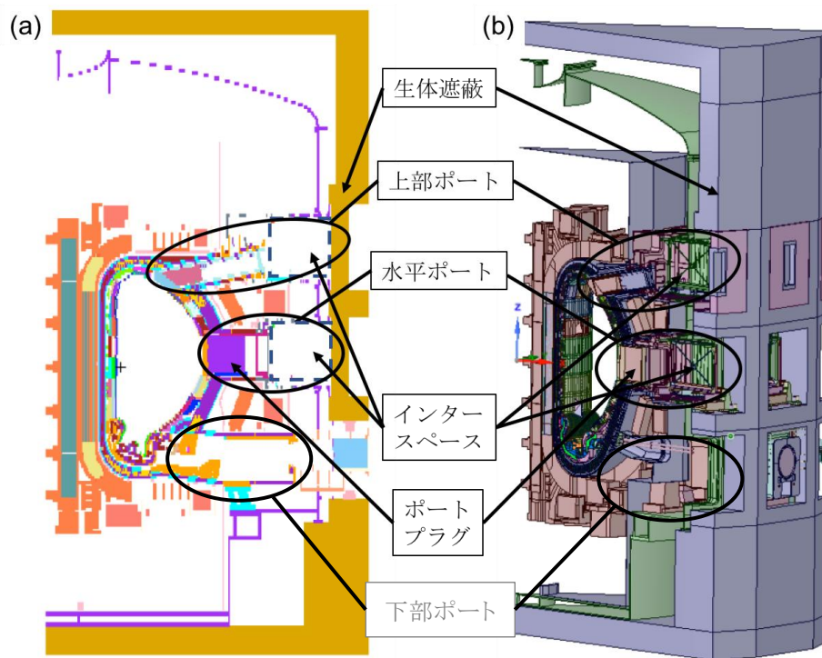
図 2.4 C-model の(a)核解析 MCNP での表示画面、(b)CAD 画像
