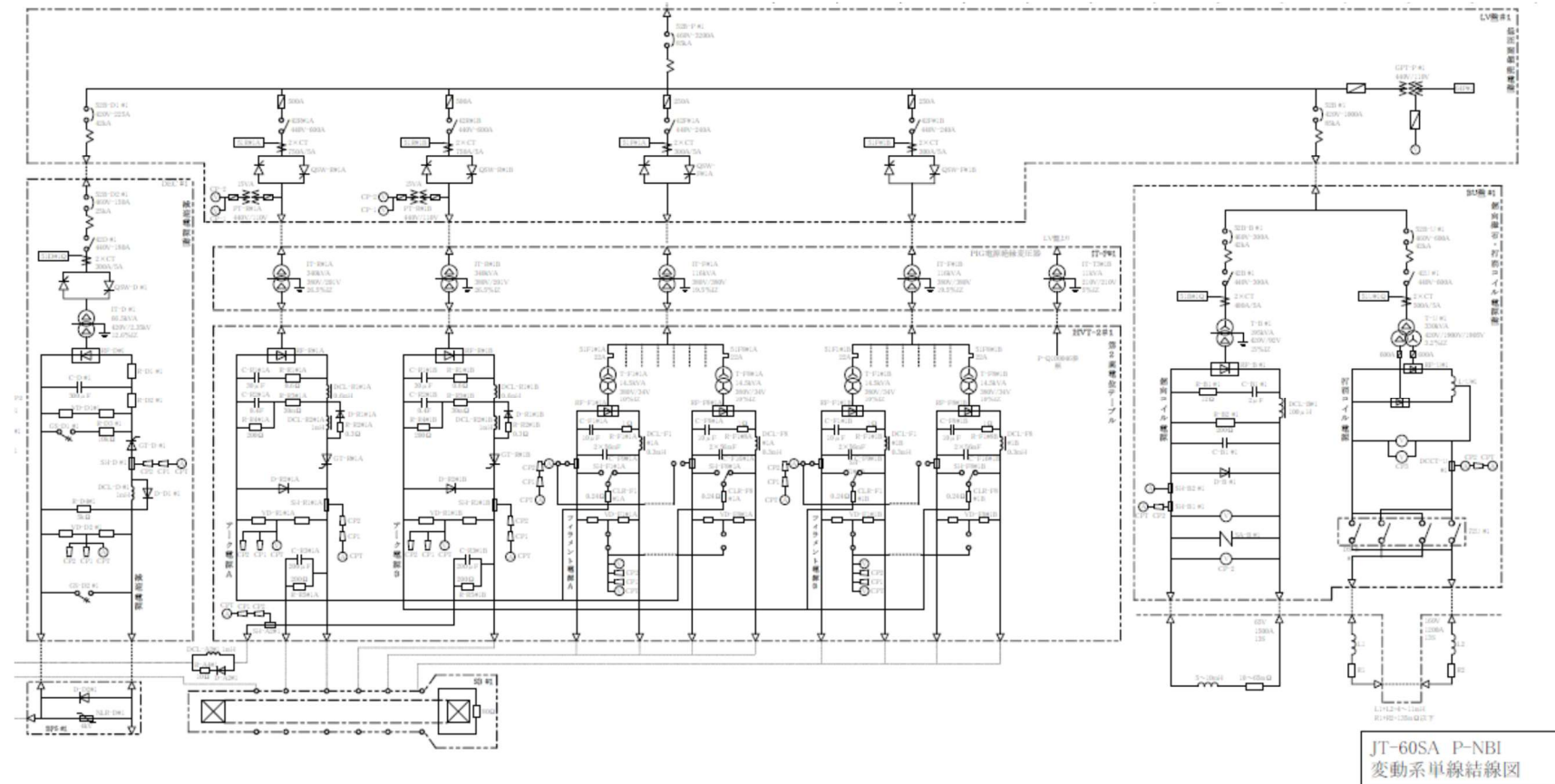
図 9 正イオン NBI 電源系配電設備単線結線図
