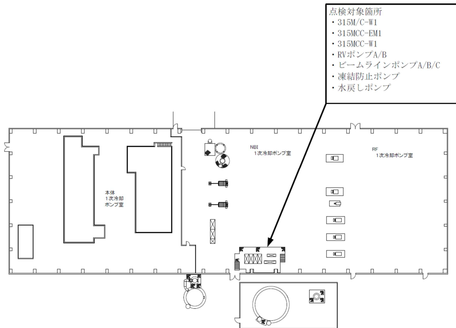
図 14 JT-60 一次冷却棟機器配置図
