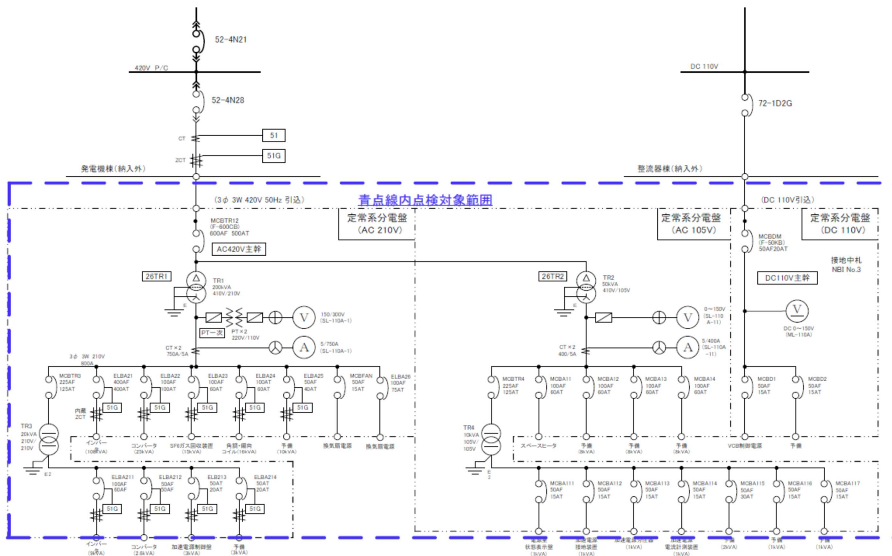
図 10 負イオン NBI 装置電源系配電設備 単線結線図
