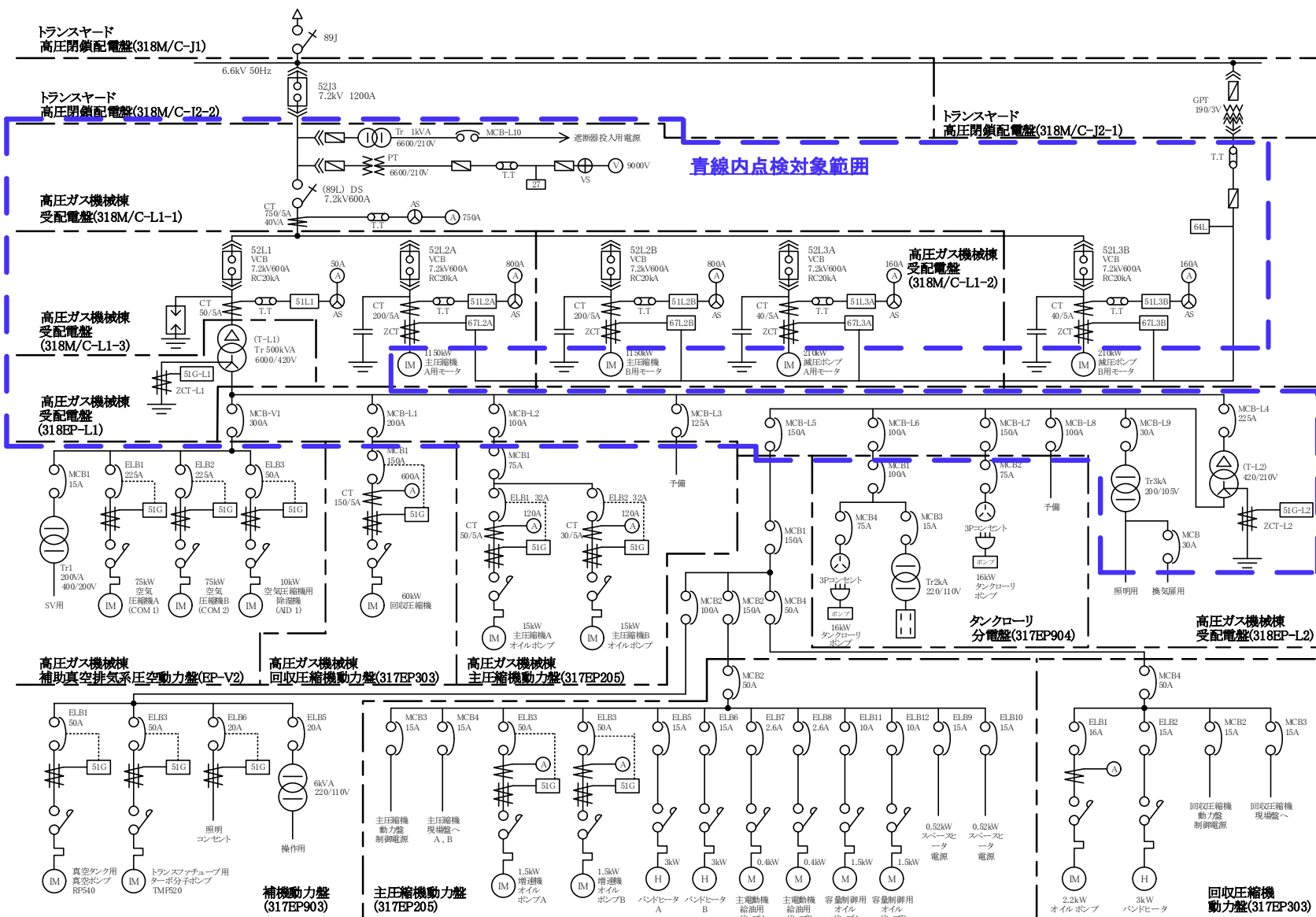
図 7 JT-60 高圧ガス機械棟受電設備及び配電設備 単線結線図
