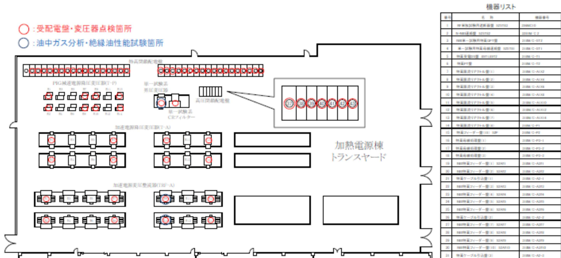
図 11 JT-60 加熱電源棟及びトランスヤード機器配置図
