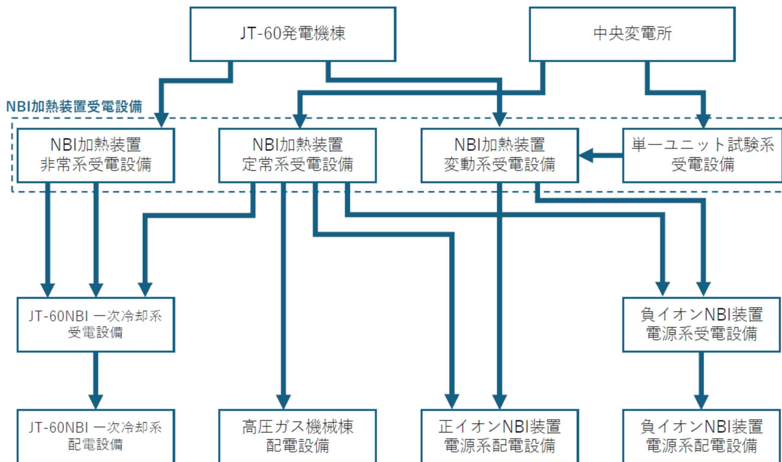
図 2 受電設備及び配電設備の系統図
