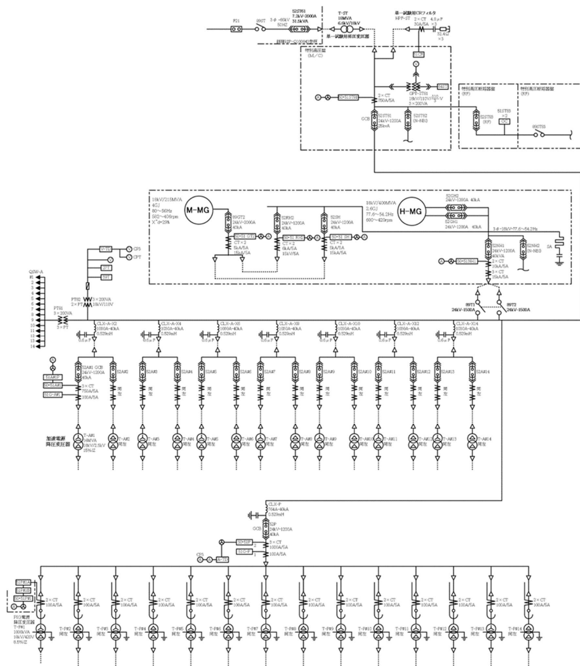
図 6 NBI 加熱装置変動系受電設備
