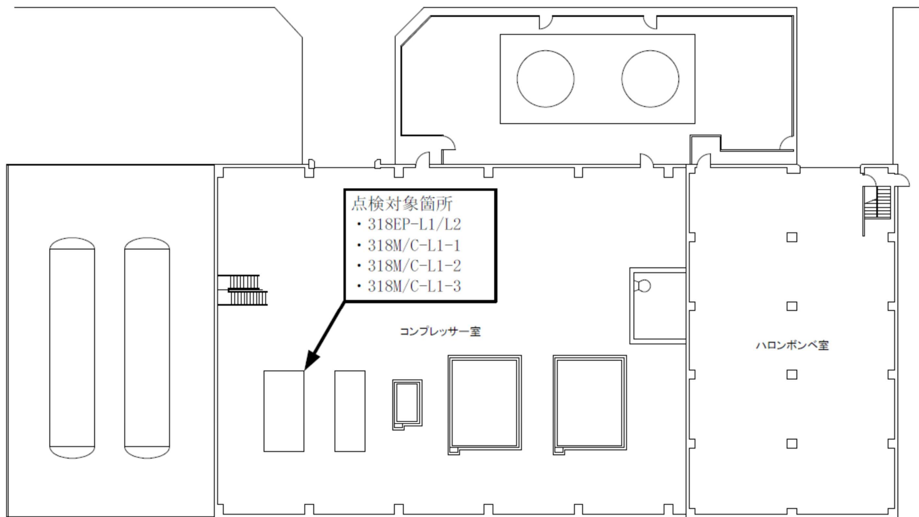
図 13 JT-60 高圧ガス機械棟機器配置図
