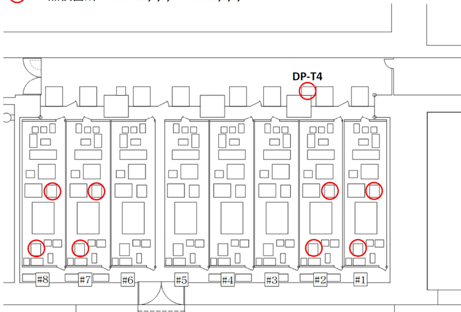
図 16 JT-60 実験棟 RV ( I ) 室機器配置図
