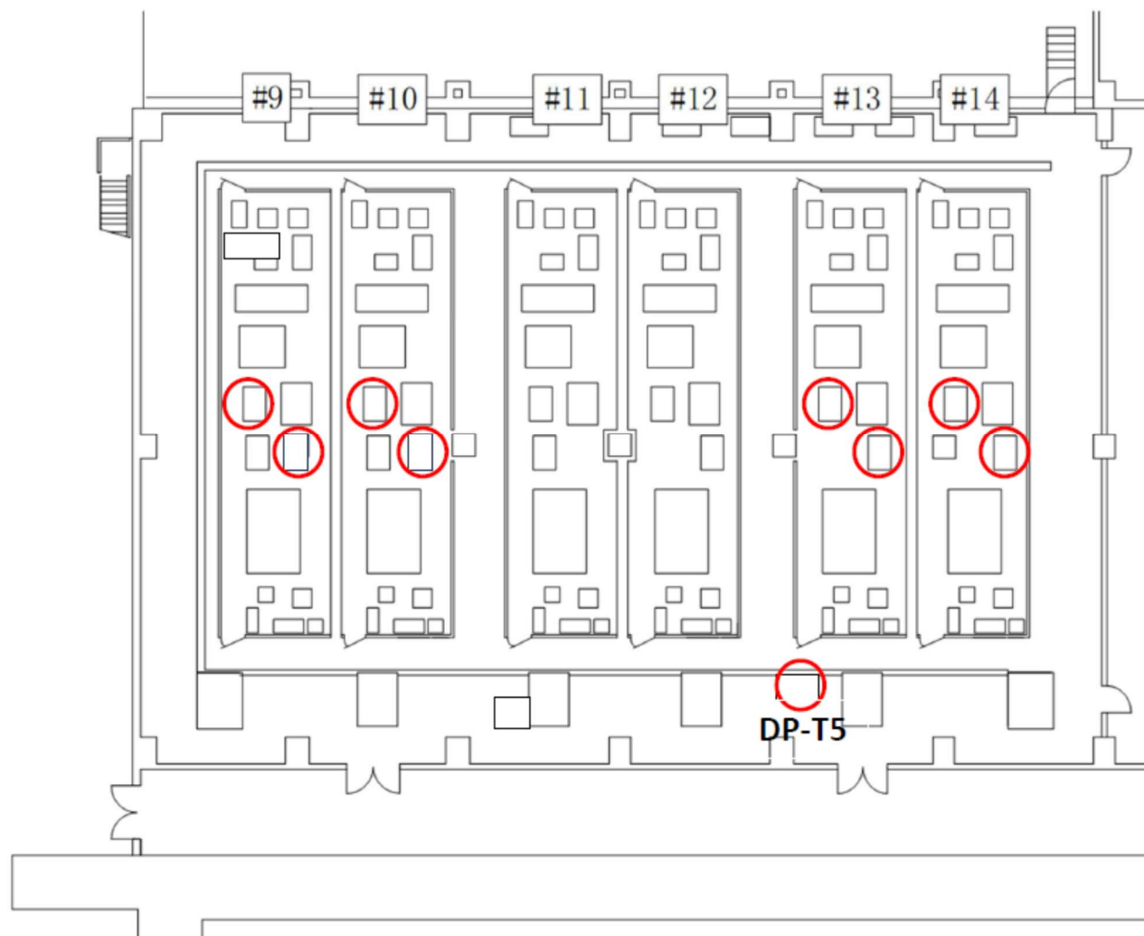
図 17 JT-60 実験棟 RV (II) 室機器配置図
