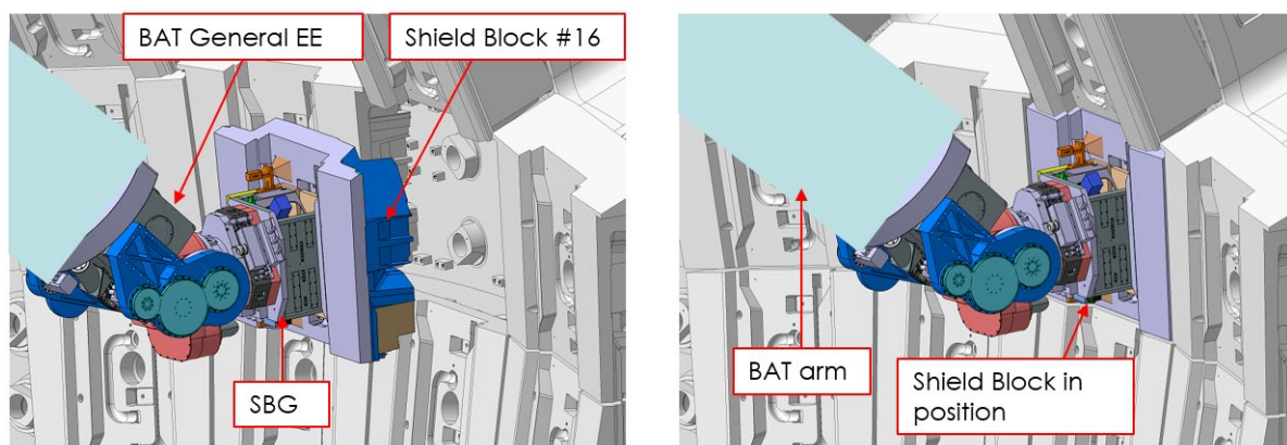
図 13 SBG プロトタイプによる SB の把持概念
