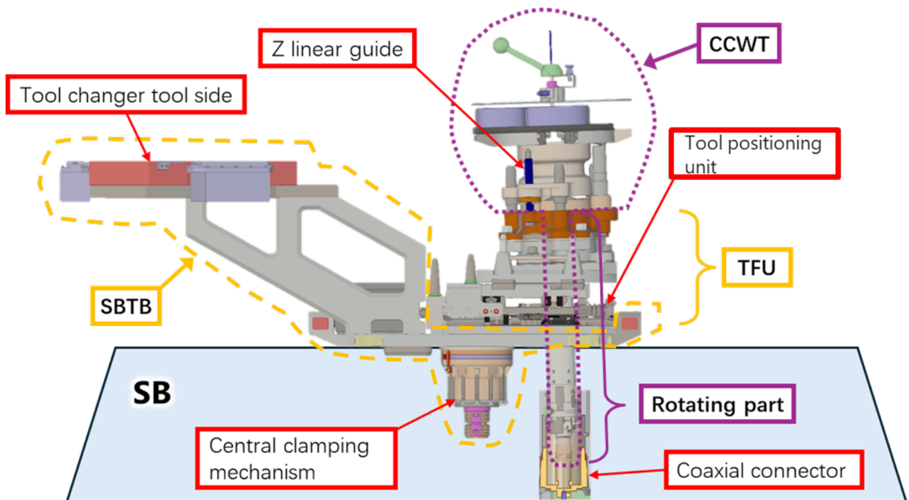
図 9 SBTB 設置手順概念図
