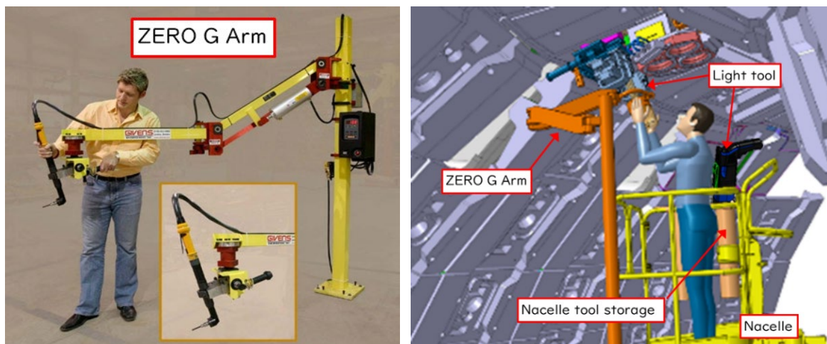
図 20 ゼロ G アームのナセル上における使用例
