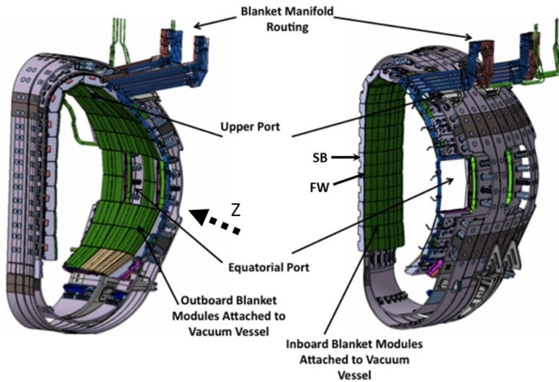
図 1 VV 内 BM 構成
