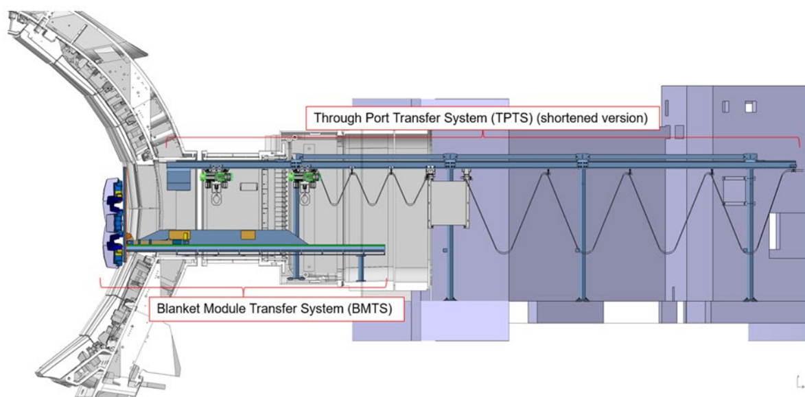
図 16 TPTS における BMTS の位置関係を示す鳥瞰図
