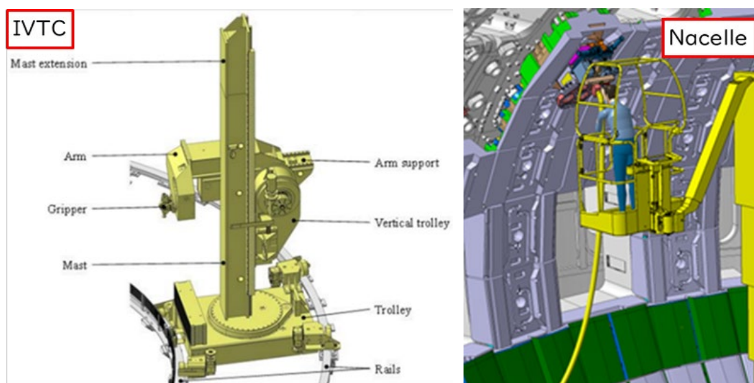
図 18 IVTC とナセル
