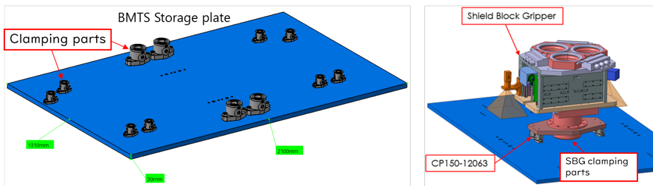
図 17 BMTS 収納板 (Storage plate)
