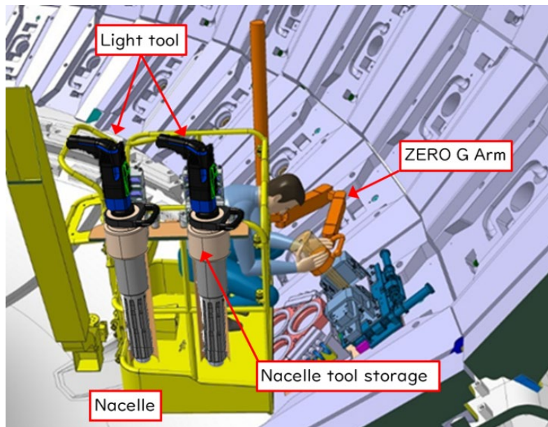
図 19 ナセル上のナセルツール収納部
