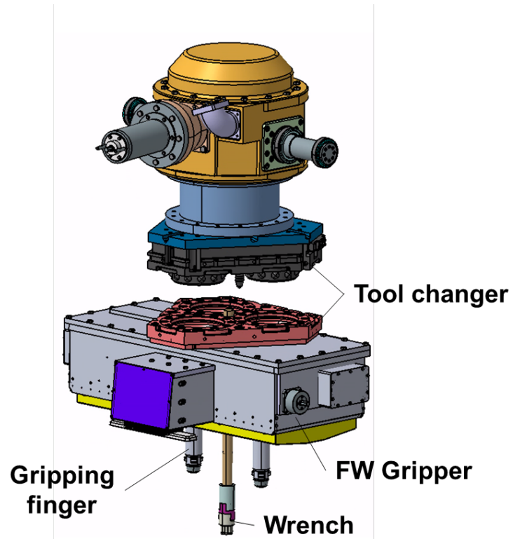
図 5 ツールチェンジャーの外観と接続イメージ (図は FW Gripper)
