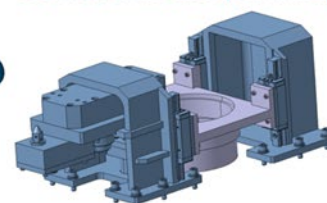
図 11 SBTB プロトタイプ及び CCWT のモジュール構成図
