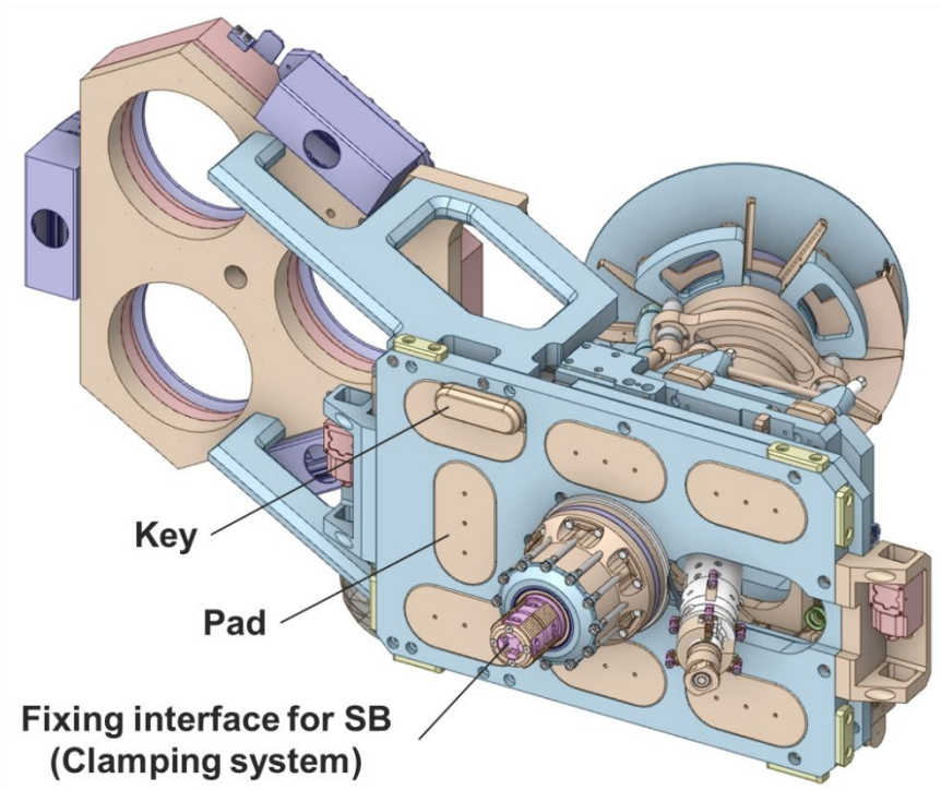
図 10 SBTB プロトタイプの概念設計
