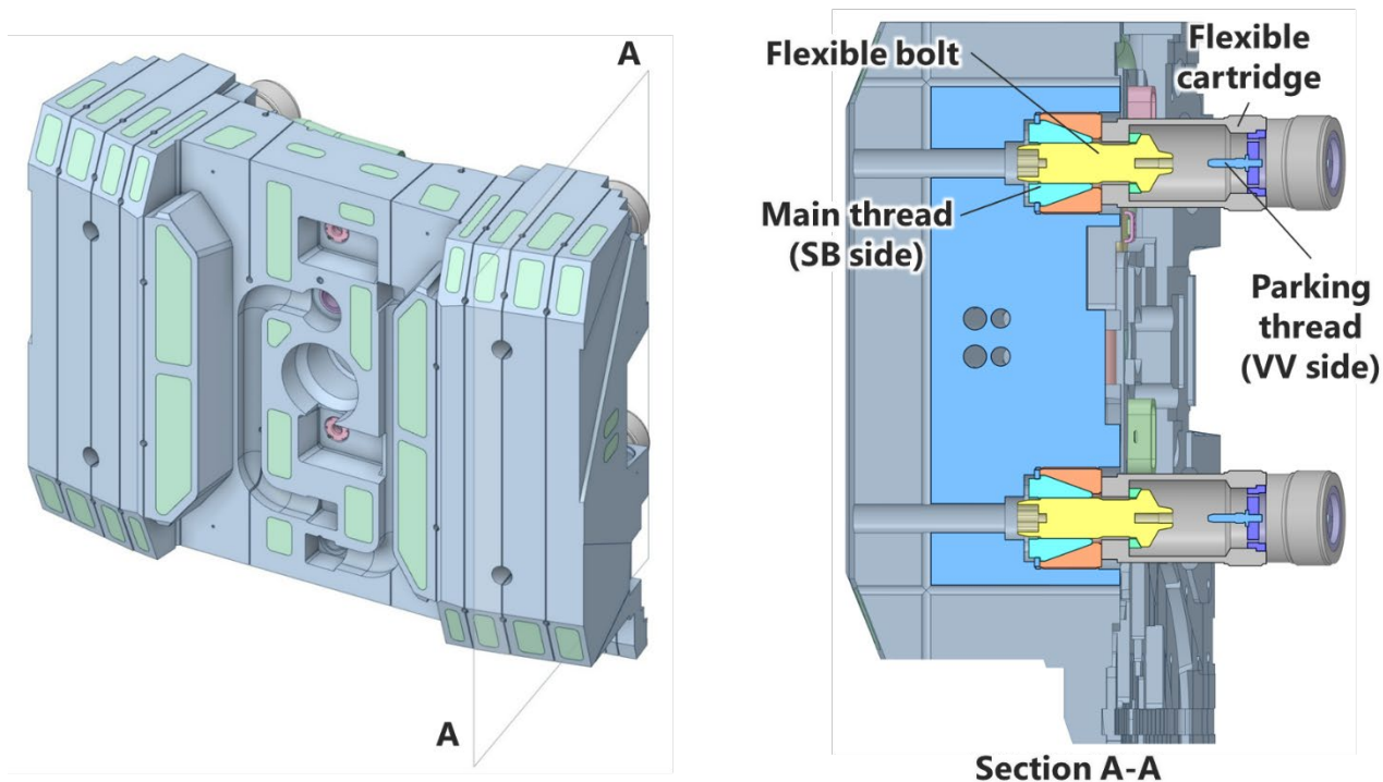
図 4 FB 部の断面図
