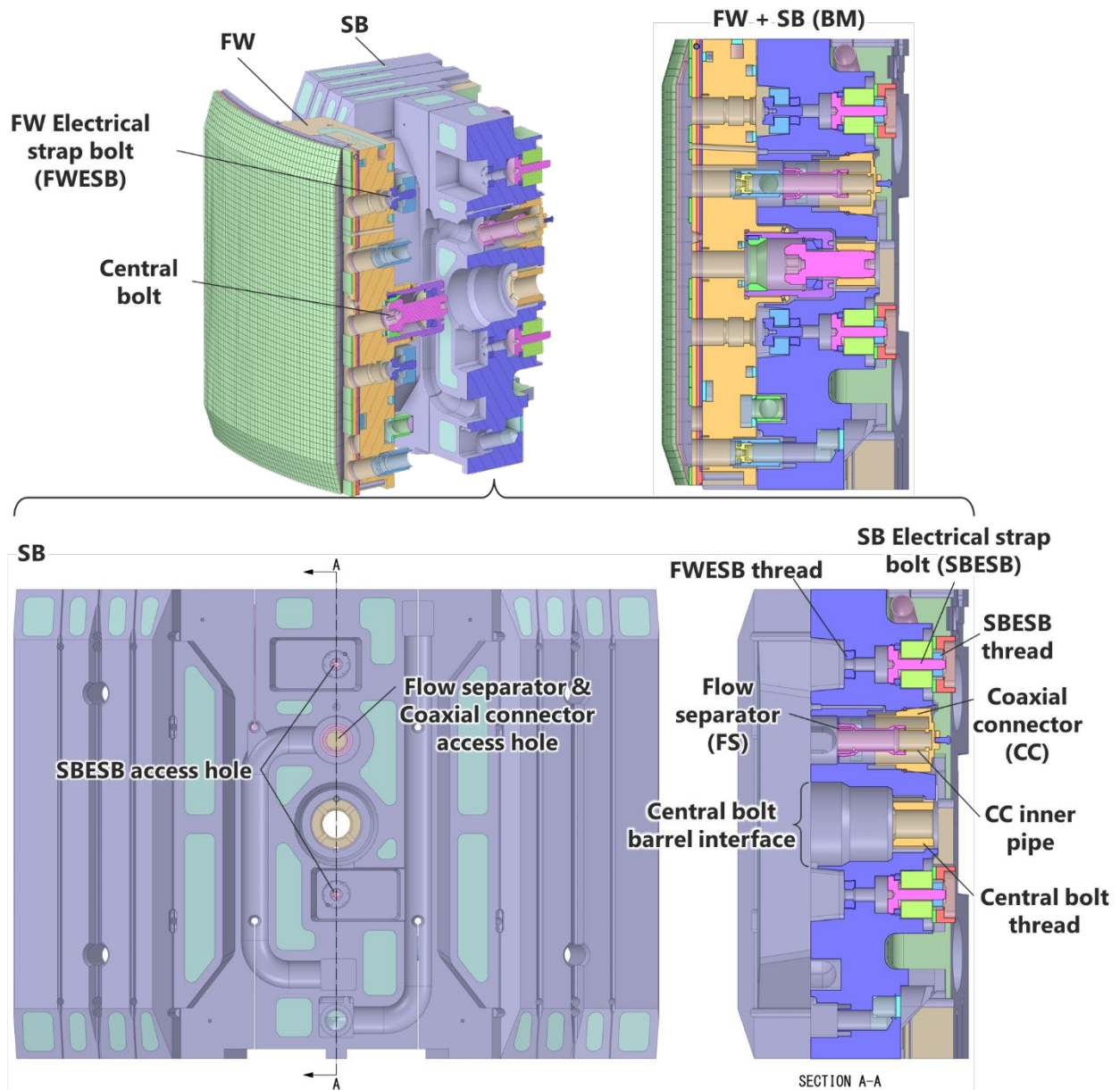
図 3 BM 構造図 (上は FW を SB に設置した状態)
