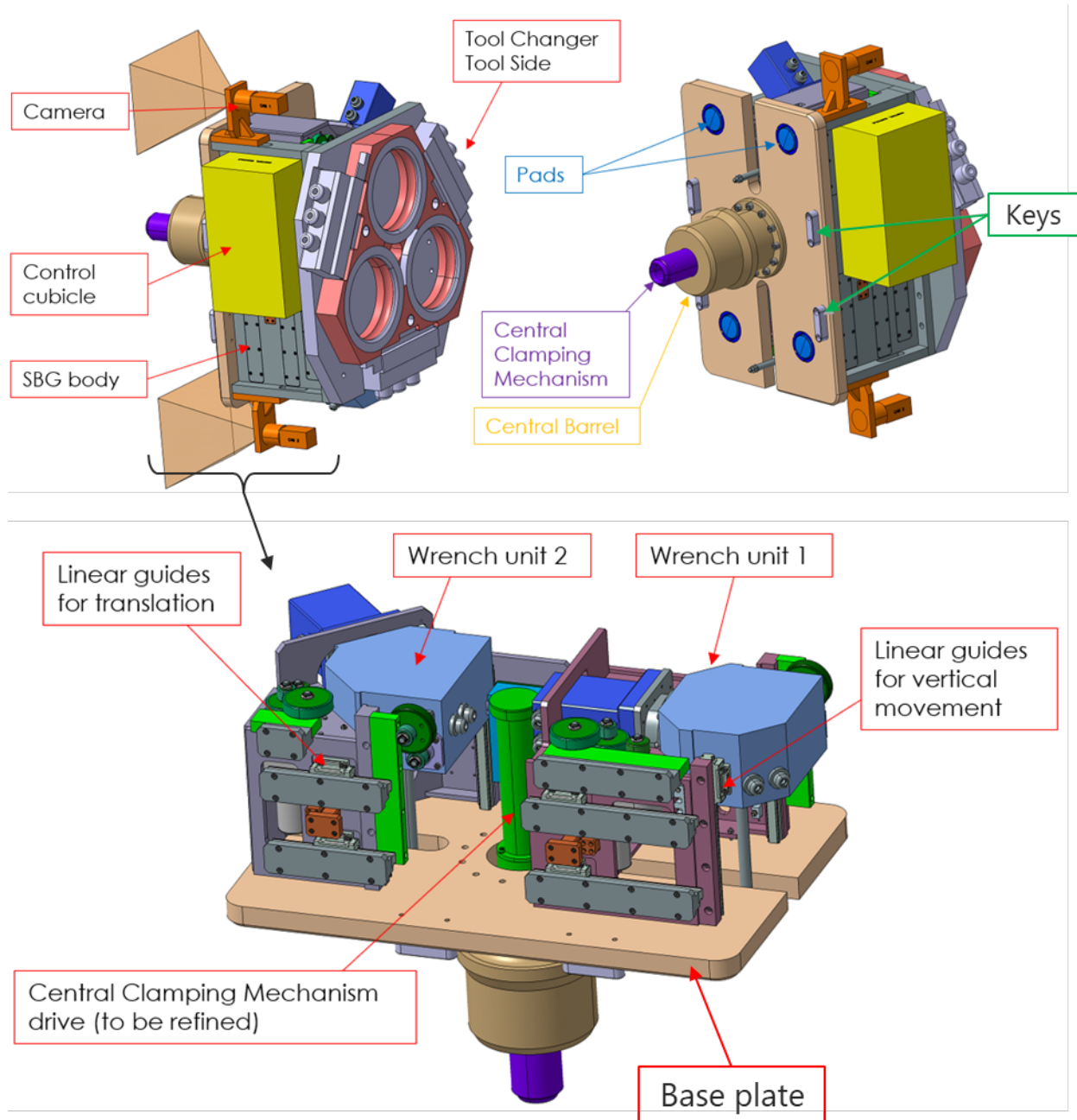
図 12 SBG プロトタイプ の概念設計
