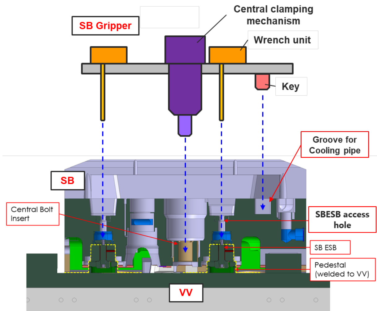
図 14 SBG プロトタイプと SB の取合い構造
