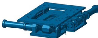
図 11 SBTB プロトタイプ及び CCWT のモジュール構成図
