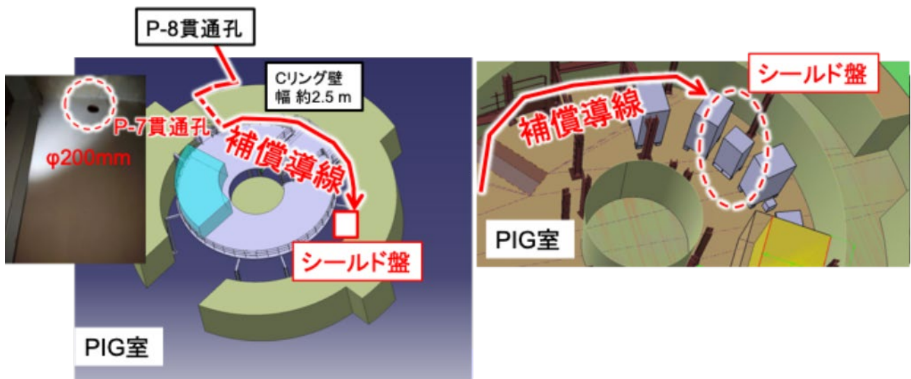
図 4. PIG 室内の P-8 貫通孔からシールド盤までのルート
