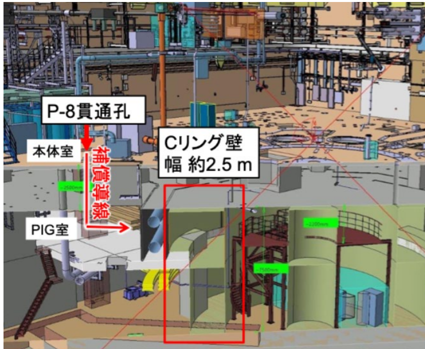
図 3. P-8 貫通孔から PIG 室までのルート
