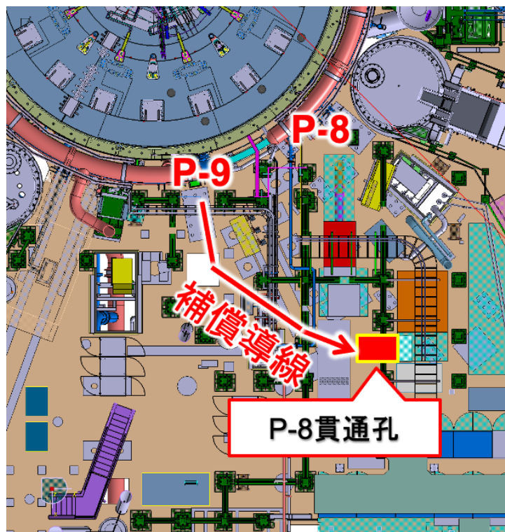
図 2. 本体室 P-9 付近から P-8 貫通孔までのルート
