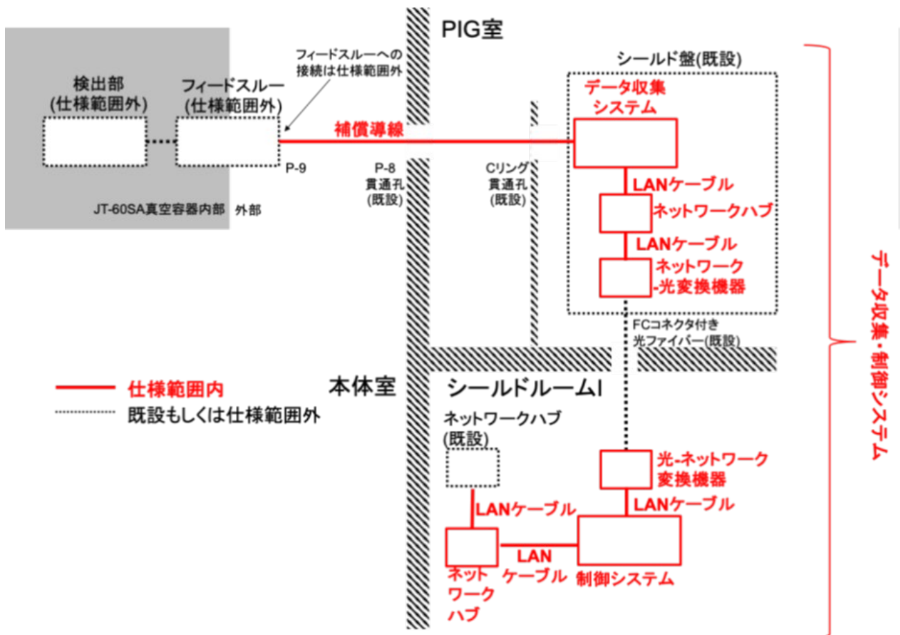
図1. カロリメータ装置全体の概要
