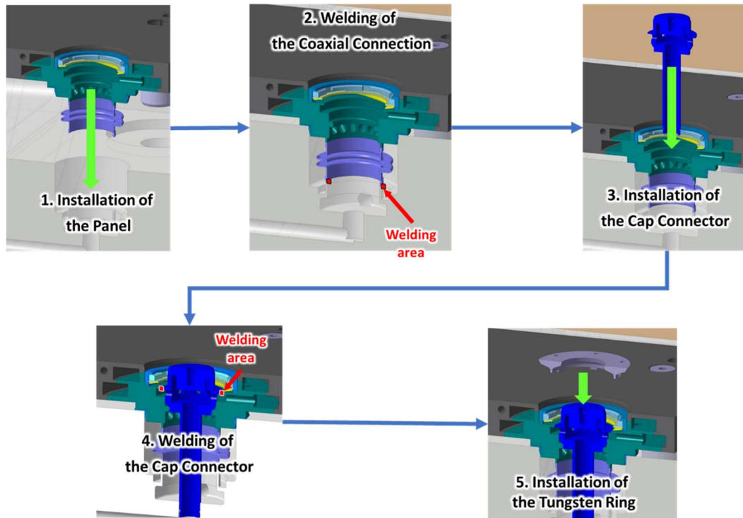
図 6 NBDL パネル取り付け作業時の冷却水配管接続箇所の溶接工程
