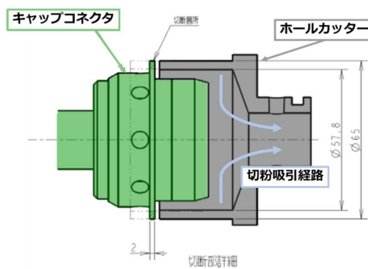
図 19 ホールカッター概形
