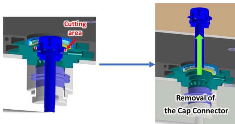
図 17 キャップコネクタの切断
