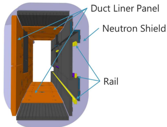
図 2 ビームポート内部（VV インボード側から見た図）
