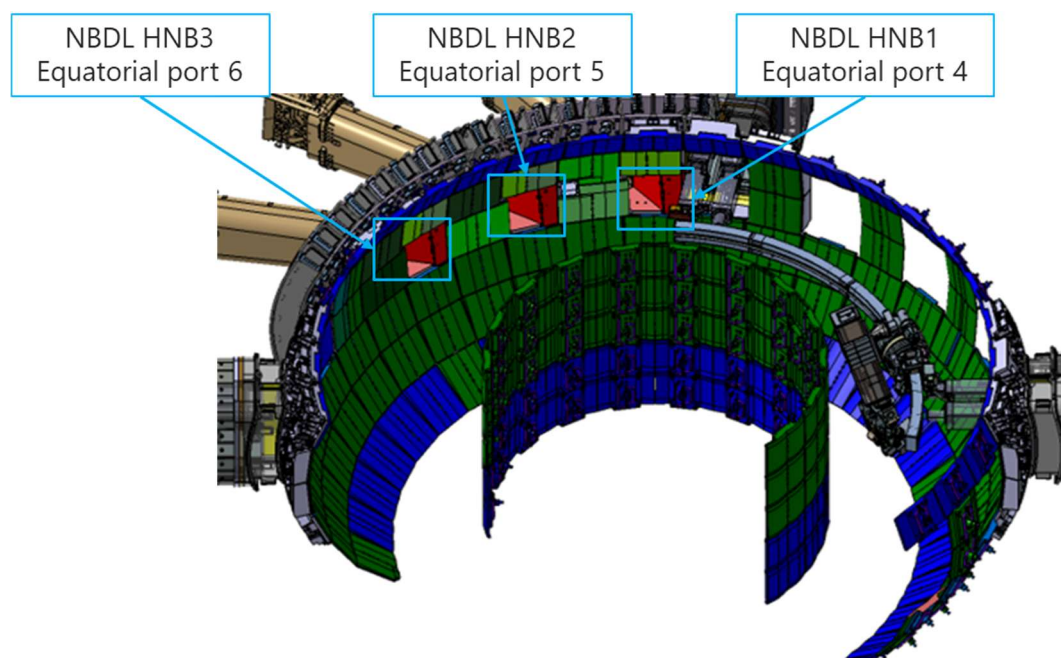
図 1 ITER 真空容器における保守対象の NBDL 位置
