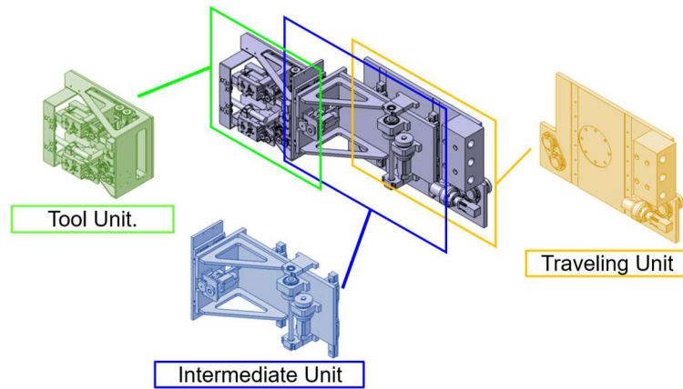
図 7 NBDL 遠隔保守装置の基本構成
