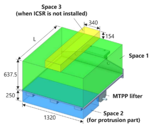
図 16 ICSR 搭載空間と MTPP 上の利用可能空間
