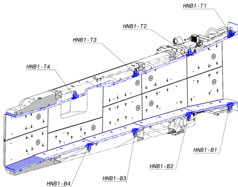
図 2 ビームポート内部（VV インボード側から見た図）
