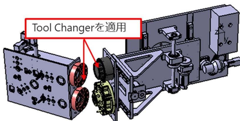
図 12 NBDL 遠隔保守装置へのツールチェンジャー適用概念図（円筒の組数を 2 組に低減）
