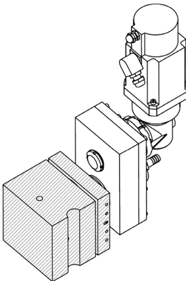
図 18 キャップコネクタ切断対象部
