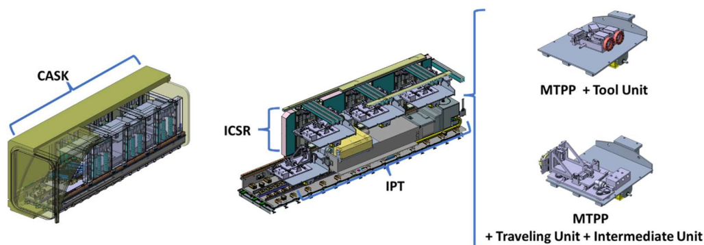
図 13 ICSR への NBDL 遠隔保守装置類の搭載概念図
