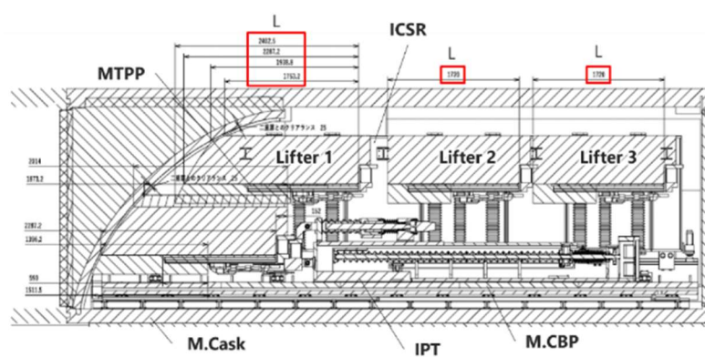
図 16 ICSR 搭載空間と MTPP 上の利用可能空間
