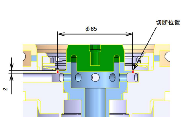
図 18 キャップコネクタ切断対象部
