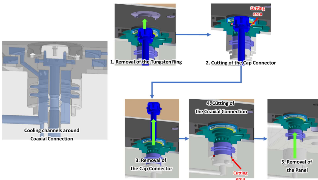
図 5 NBDL パネル取り外し作業時の冷却水配管接続箇所の切断工程
