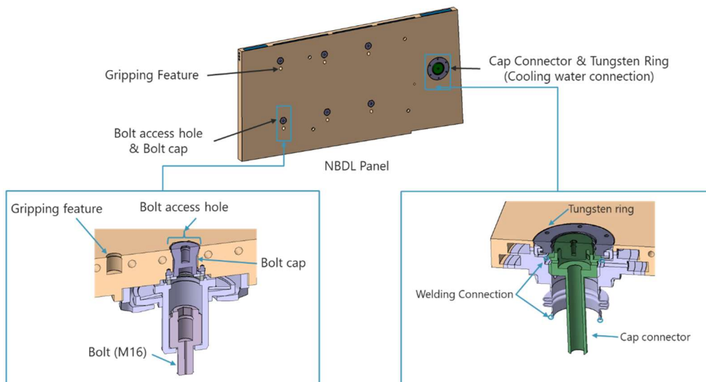
図 4 NBDL 内部構造及び NBDL パネル
