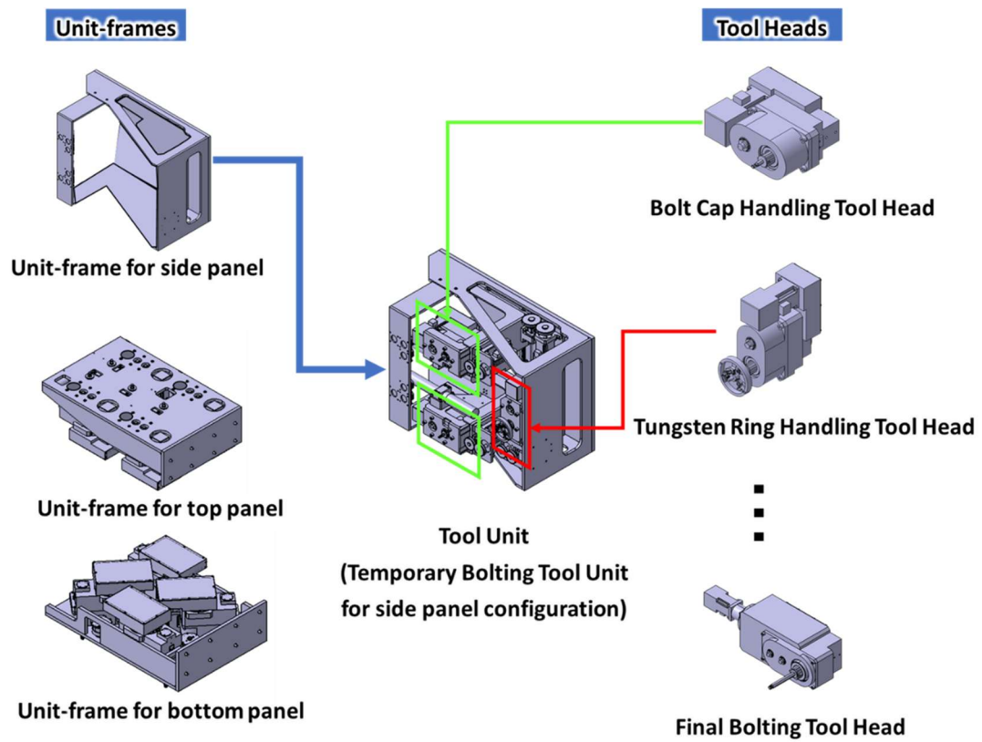
図 8 ユニットフレームとツールヘッドによるツールユニットの構成
