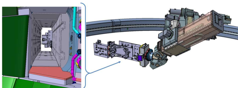
図 9 VMNP による NBDL 遠隔保守装置のビームポートへの設置時姿勢概念図
