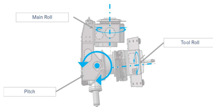
図 10 VMNP のリスト構造部の回転軸及び各名称
