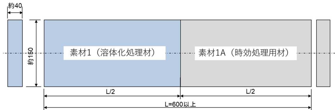
図 1. 鍛造板の分割図
