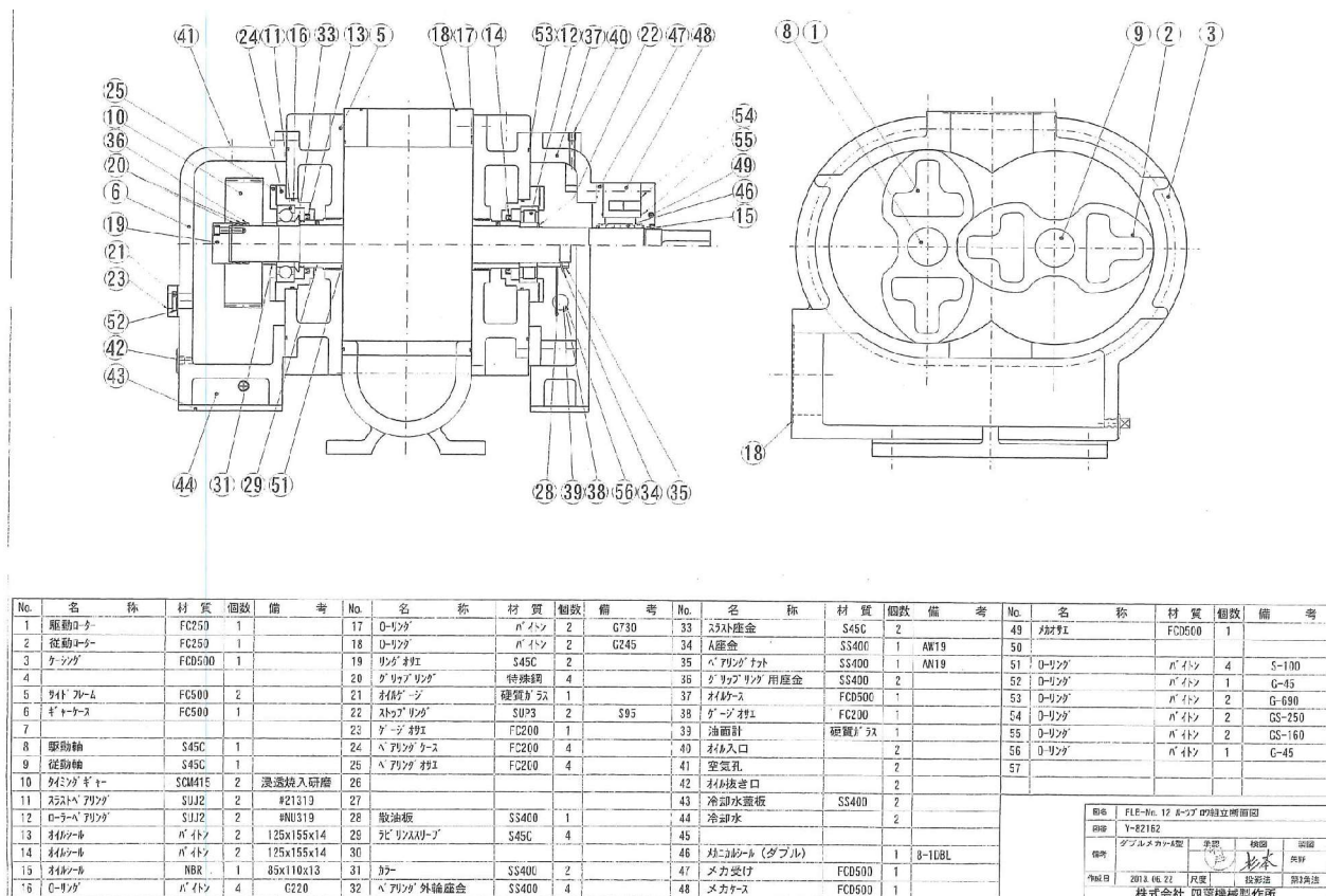
図3 ブロワ構造図
