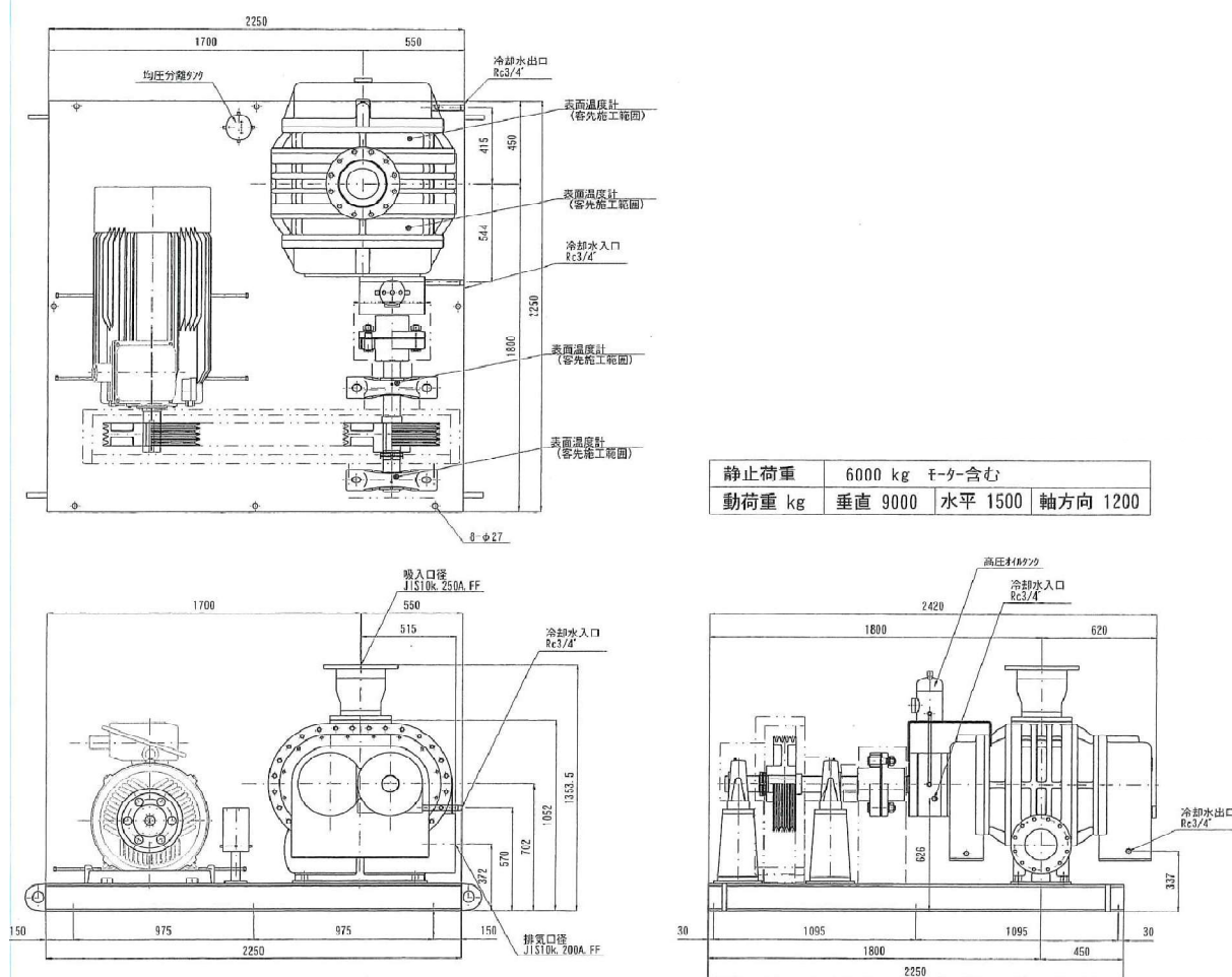
図2 ブロワ B4 外形図
