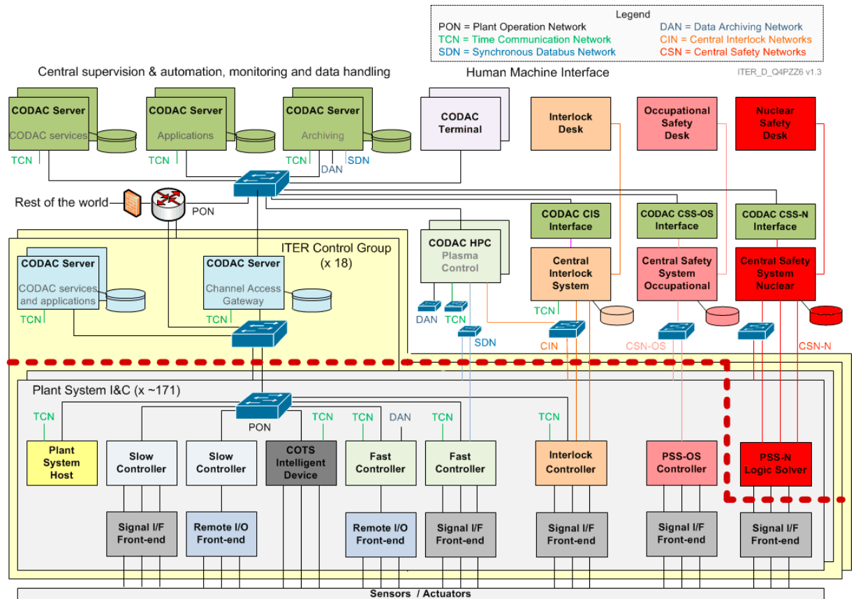
図8 イーターのPlant System I&C physical architecture
