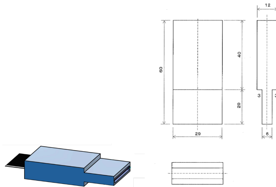
図 1：導入機コネクタ 模式図
