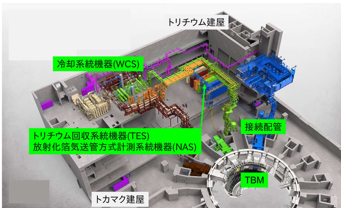
図 2 イーターに設置する TBS
