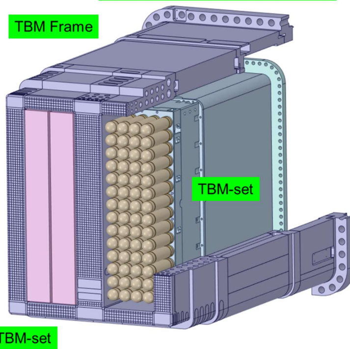
図 4 2 つの TBM-set と TBM Frame からなる TBM PP
