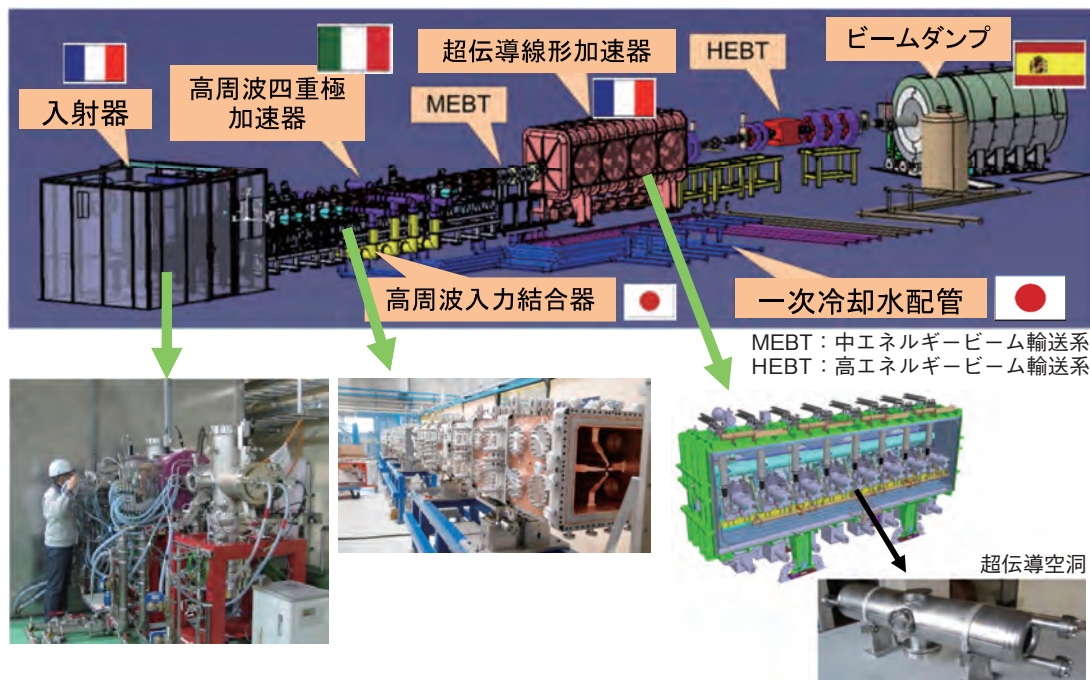
IFMIF原型加速器構成概念図
