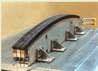
耐熱タイルの実規模試験体（全長：約1.3m）
