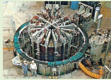
13テスラ発生に成功したITER用超伝導モデル・コイル(外径3.6m)
