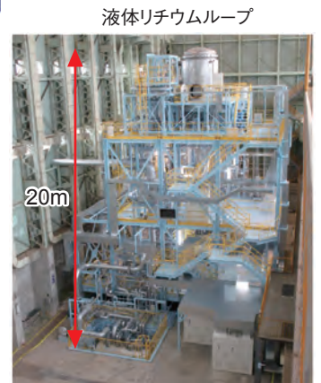
液体リチウムループ
