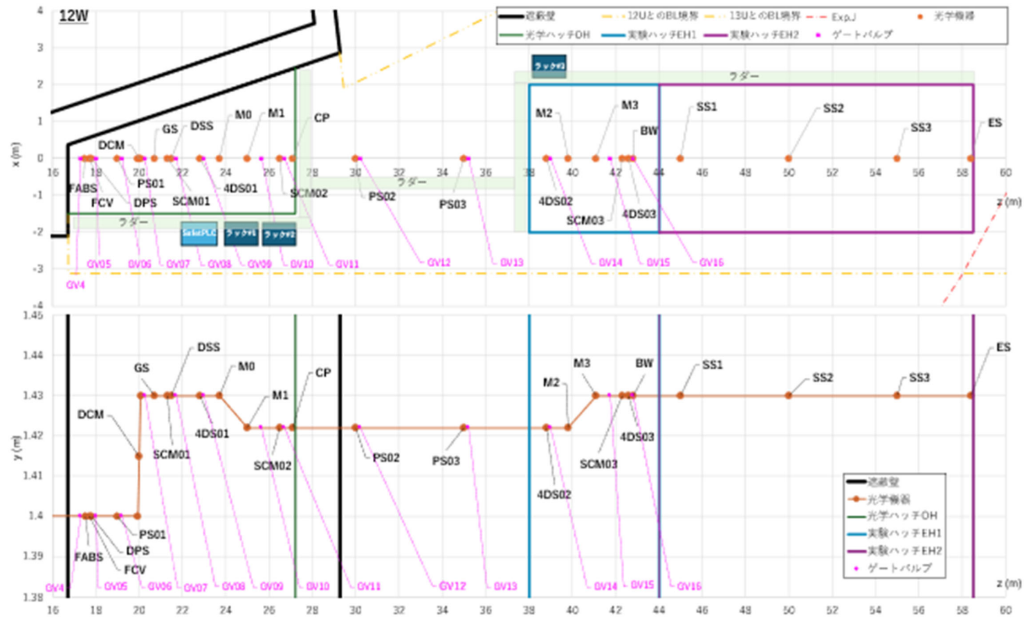
図 2 BL12W 光学機器配置図 (参考図)
