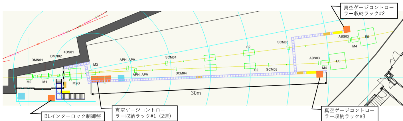
図 1 BL12U 光学機器配置図 (参考図)
