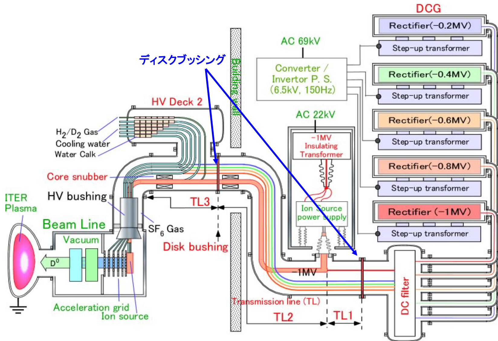
図 3 ITER NBI のシステム構成
