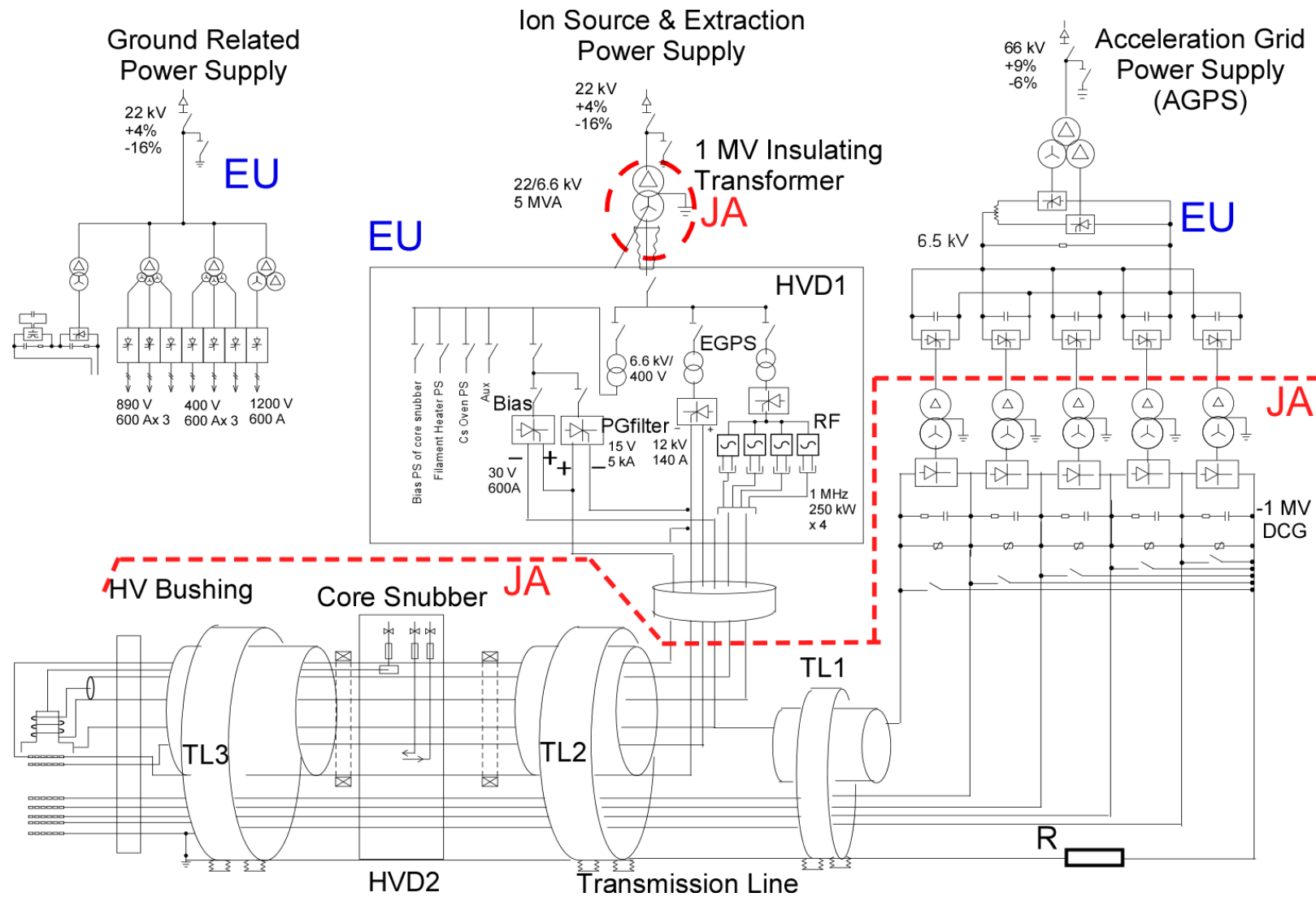
図 2 ITER NBI の電源回路
