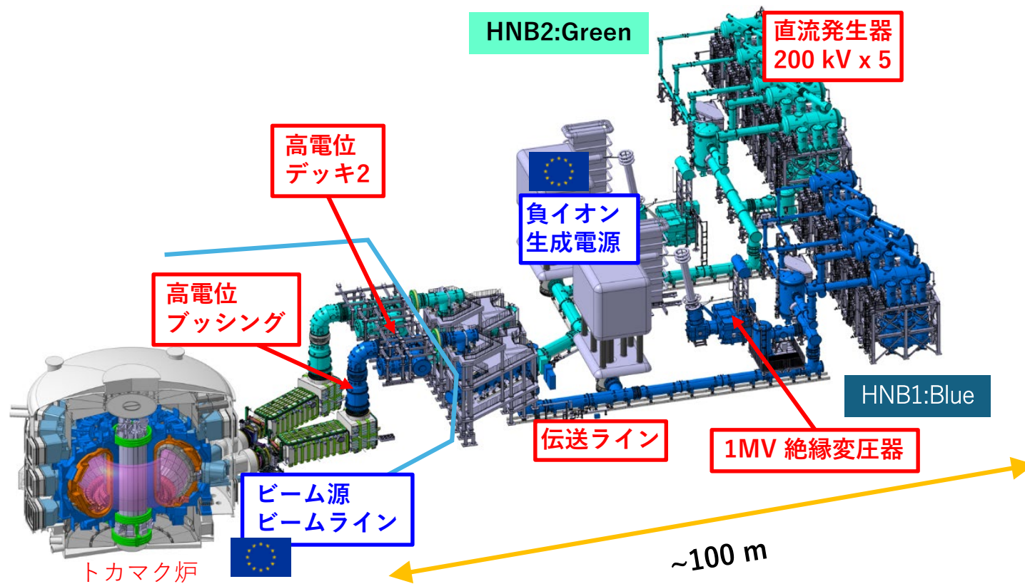
図 1 ITER NBI の鳥瞰図
