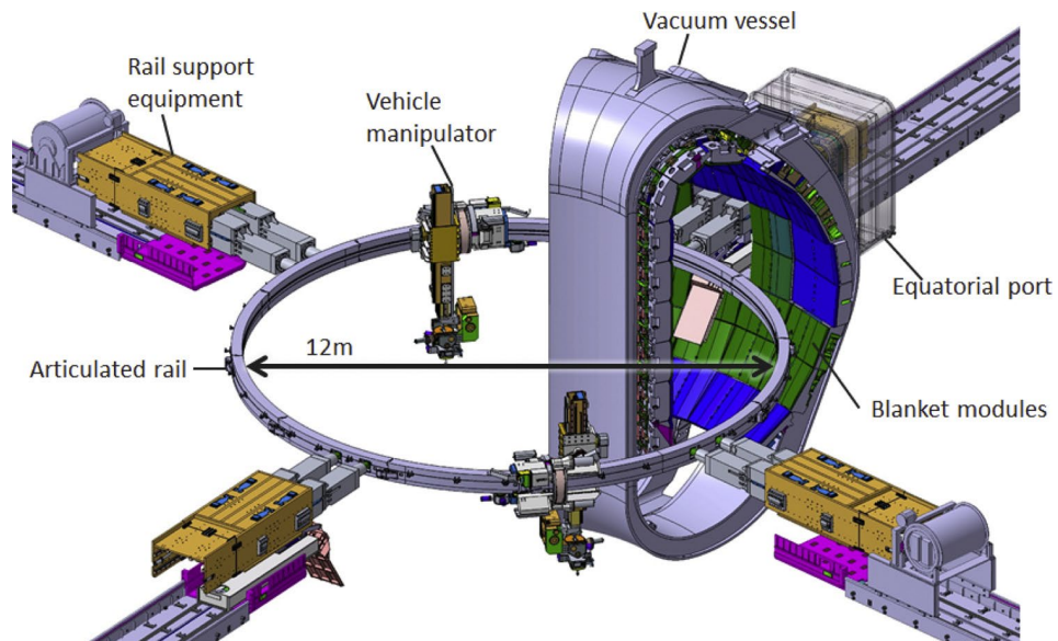
図 1 真空容器内に展開されたブランケット遠隔保守システム
