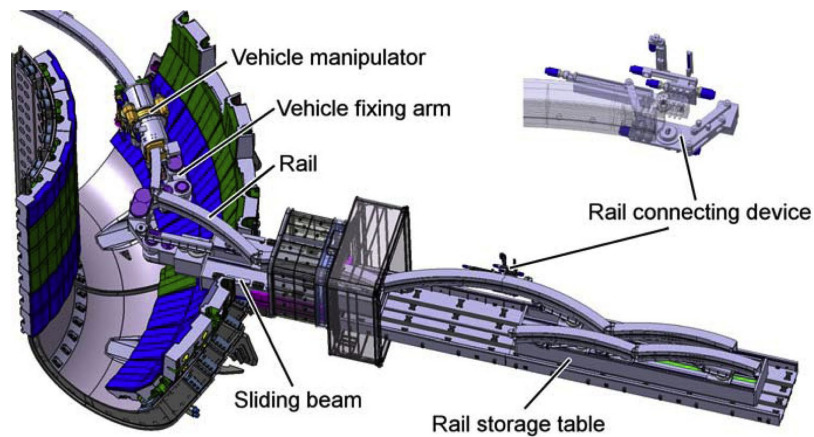
図 2 真空容器内に展開している途中のブランケット遠隔保守システムの構成
