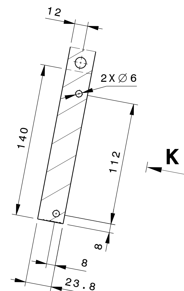
DETAIL J Scale: 1:2
