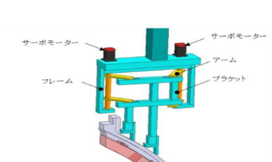
(A) 上部ポートアクセス方式
