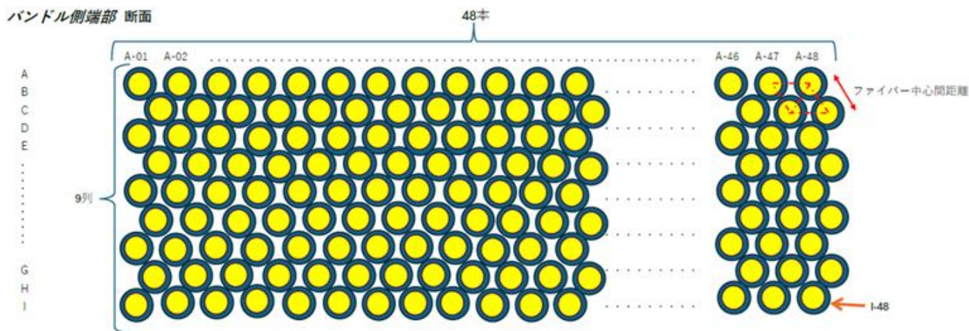
図 2.1-1 光ファイバーバンドル側端部の配列参考図
