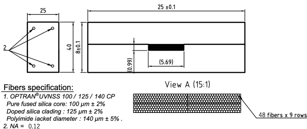
図 2.1-2 光ファイバーバンドル側端部コネクタの参考図及び寸法
