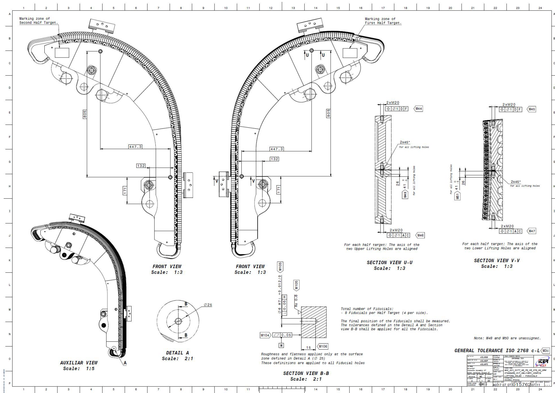
添付図 7 フル・タングステン・ダイバータ 外側垂直ターゲット (7)
