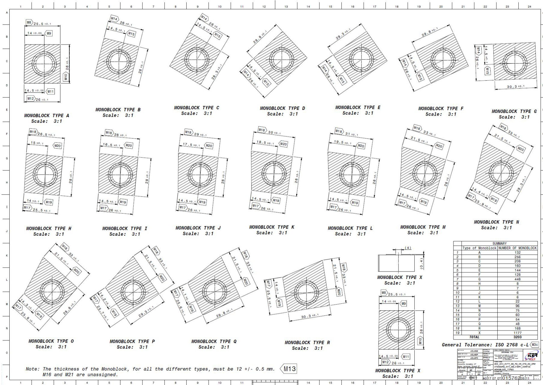
添付図 5 フル・タングステン・ダイバータ 外側垂直ターゲット (5)
