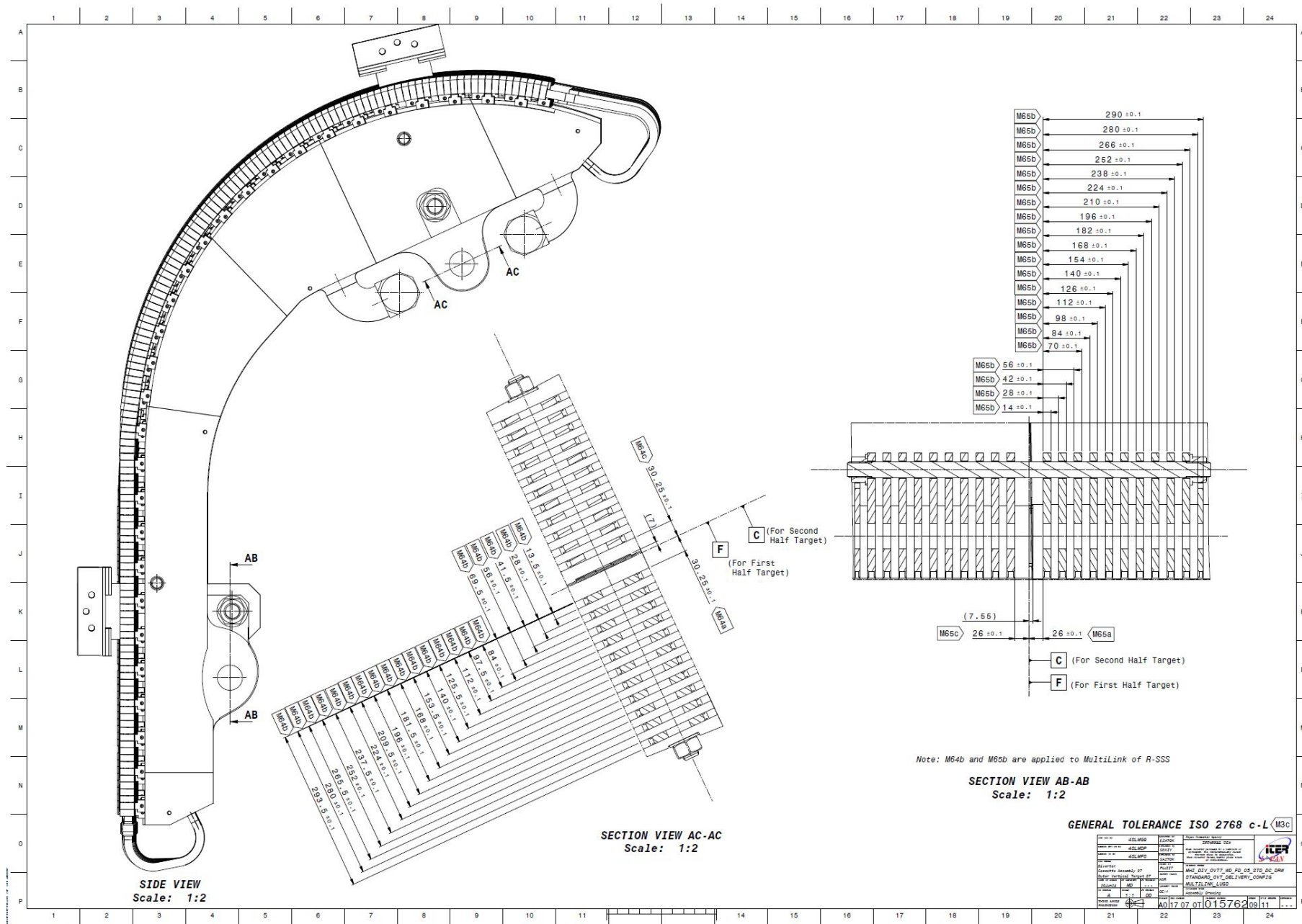
添付図 9 フル・タングステン・ダイバータ 外側垂直ターゲット (9)
