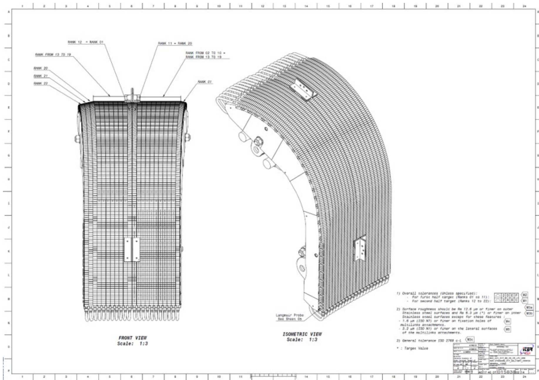
添付図 16 LPV-OVT の参考図
