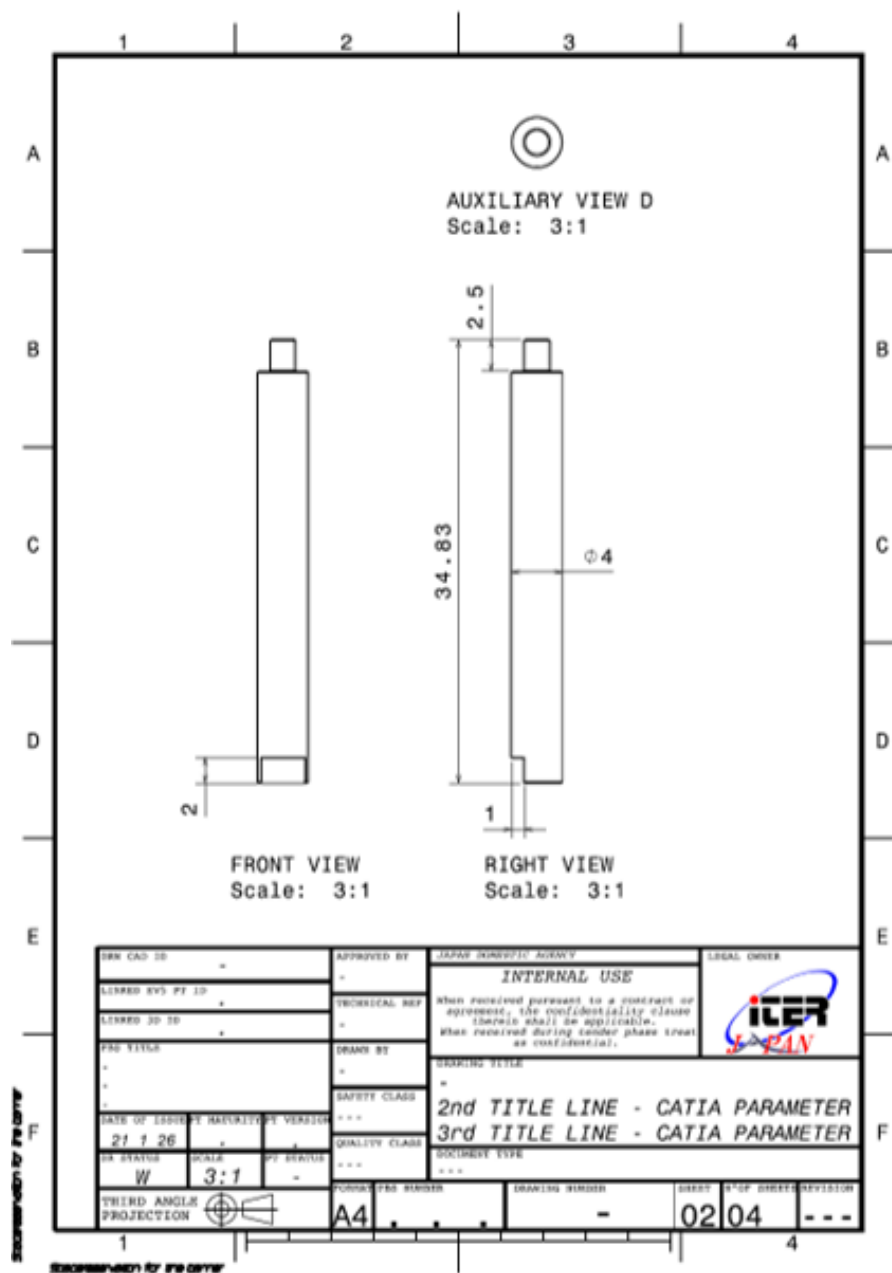
添付図 19 LP の参考図：(2)プローブ（材質 W）、(3)絶縁管（材質セラミック）
