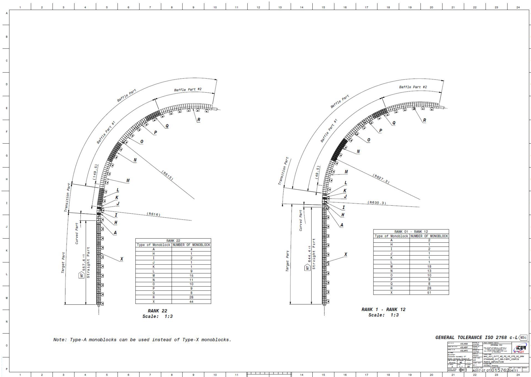
添付図 4 フル・タングステン・ダイバータ 外側垂直ターゲット (4)
