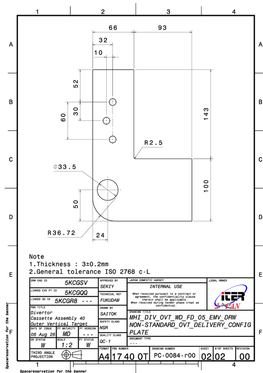
添付図 24 EMV-OVT 用下部スパーサの参考図
