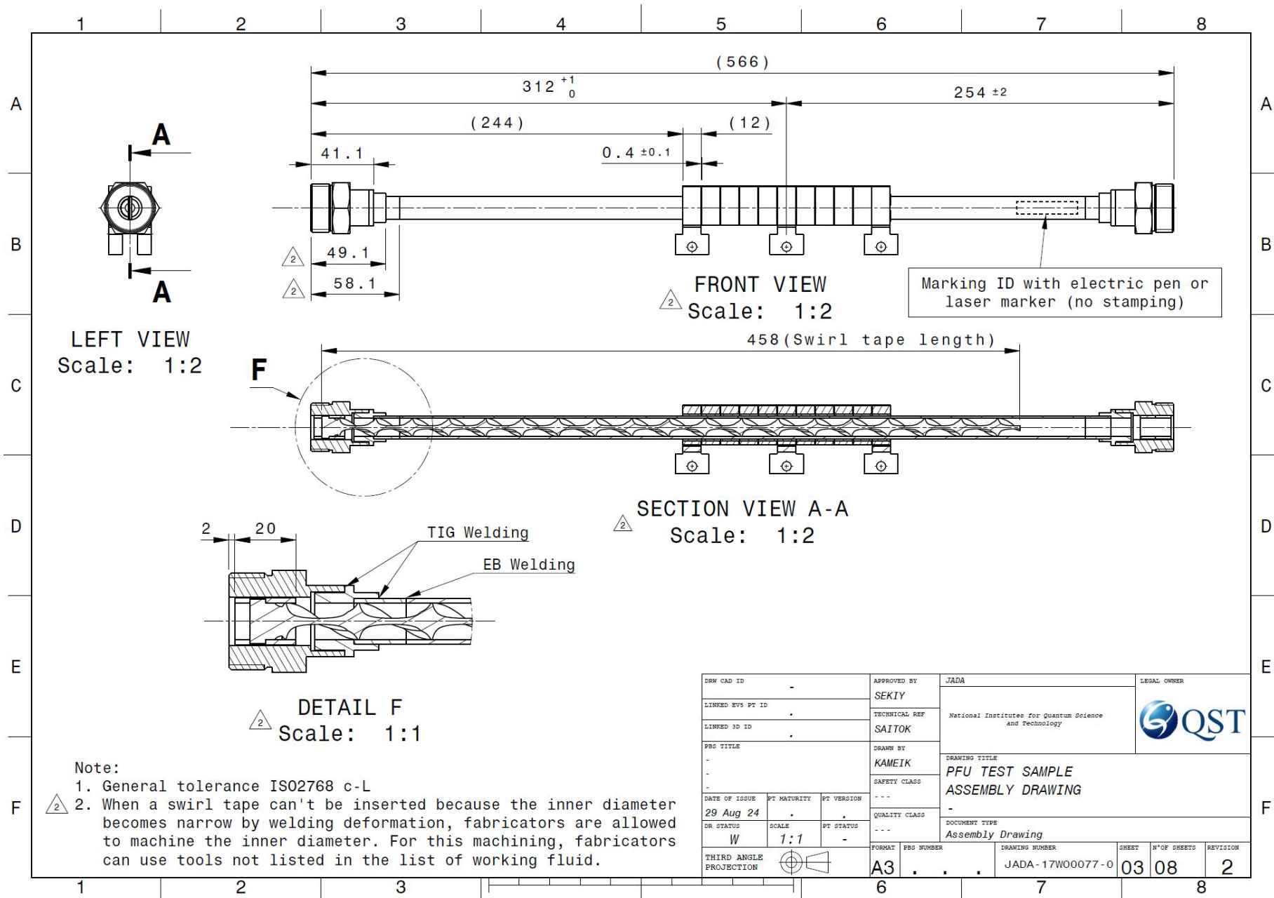
添付図 13 OVT PFU テストサンプル 概念図
