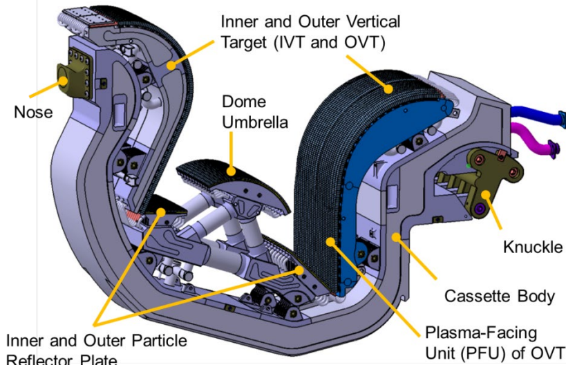
Figure 1.2-1: 3D view of the ITER W Divertor. / 図 1.2-1: ITER W ダイバータの 3D 図
