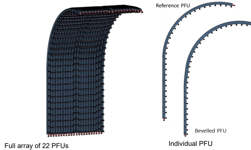
Figure 4.1-2: schematic 3D view of the PFU. /図 4.1-2: PFU の概略 3D 図
