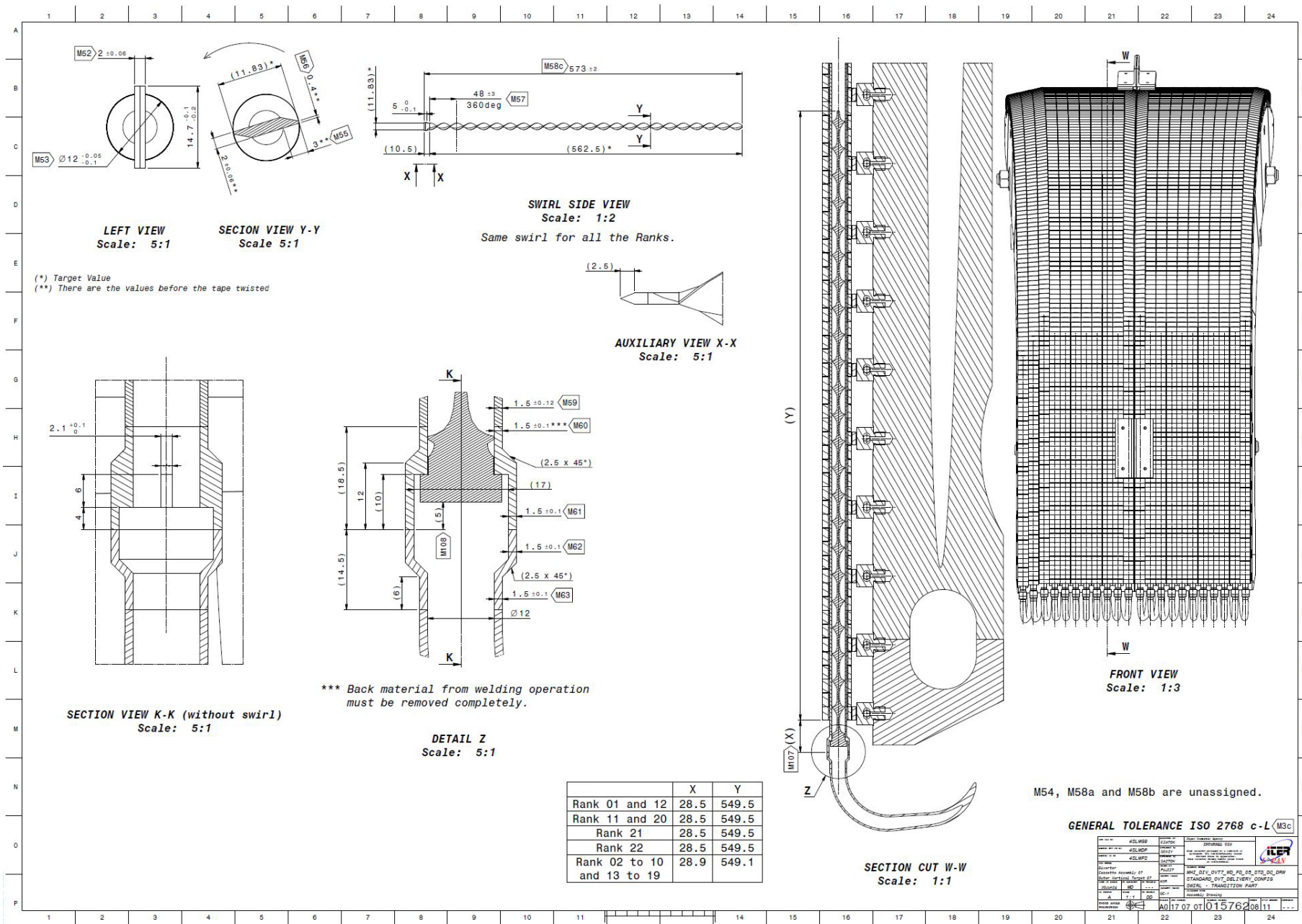
添付図 8 フル・タングステン・ダイバータ 外側垂直ターゲット (8)
