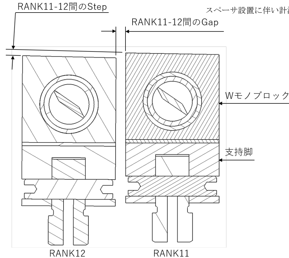
添付図 23 OVT 組合せ試験における RANK11 及び RANK12 の Gap 及び Step の参考図。
