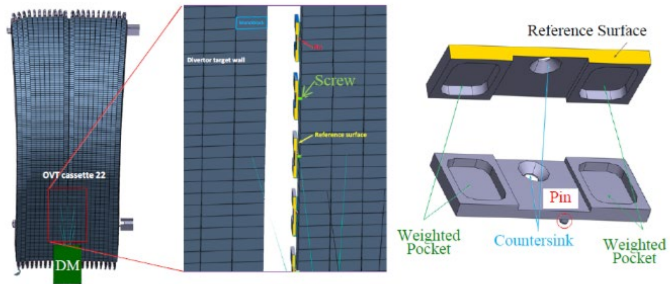
添付図 21 EMV-OVT の参考図
