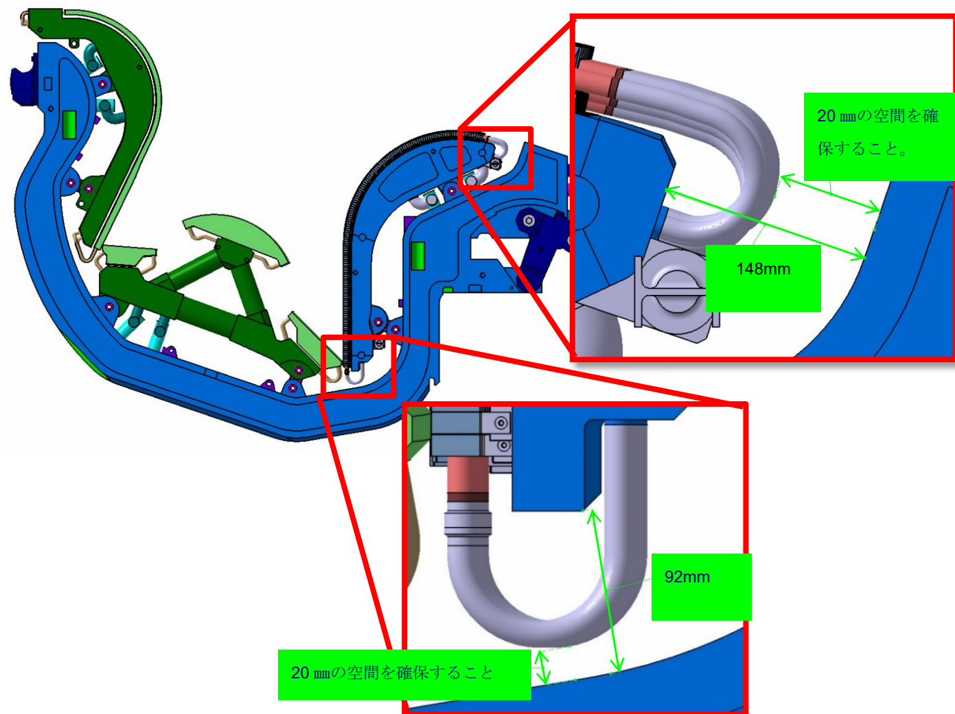
添付図 12 PFU-SSS 接続配管と CB の位置関係 参考図
