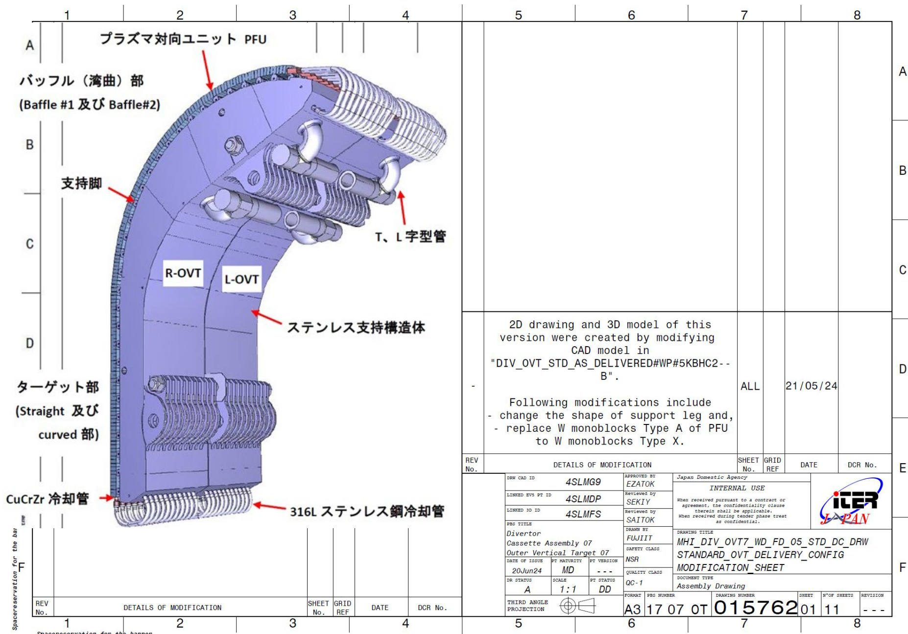
添付図 1 フル・タングステン・ダイバータ 外側垂直ターゲット (1)
