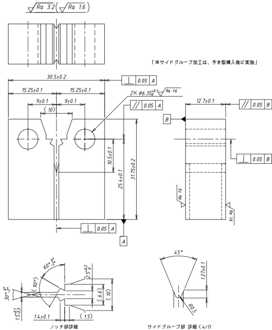
図 2.1 破壊靱性試験片の概略
