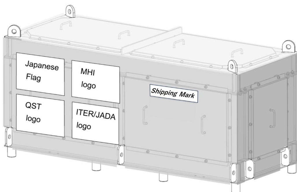
図2 輸送品（OVT 本体）の引き渡し時の外観概略図。輸送品はオーニングシートで覆われている オーニングシートには輸送品である内容物の説明紙、Shipping Mark, 日本の国旗、製作者の ロゴ、QST のロゴ、ITER 国内機関（JADA）のロゴが、片面に貼りつけられている。
