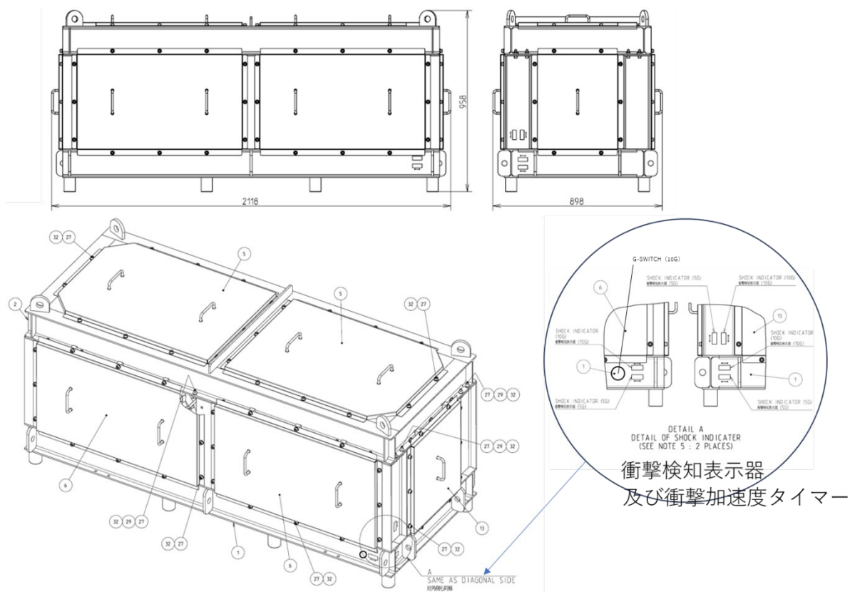
図1 輸送品 (OVT 本体) の参考図 (ITER ダイバータ外側ターゲットを輸送容器に設置した状態)。 輸送架台には、衝撃検知表示器 (5G 及び 10G) を 3 方向に各 2 か所 (計 12 個)、衝撃加速度 タイマー (10G) を対角位置に各 1 か所 (計 2 個) 設置している。
