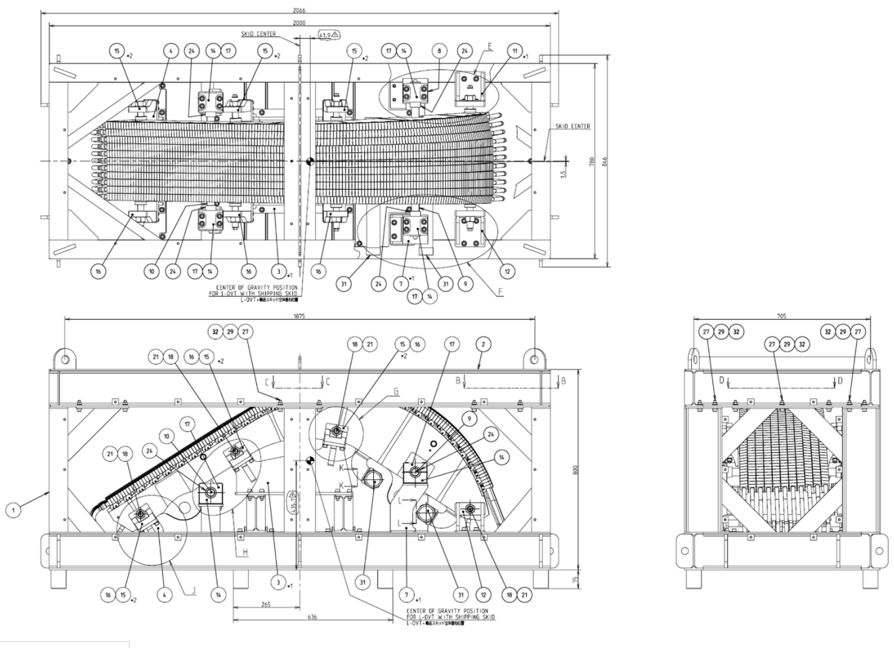
図3 輸送品（OVT 本体）の重心位置（輸送容器の外装パネルとオーニングシートは非表示としている）。ITER ダイバータ外側ターゲットは、輸送容器の中に設置されている。
