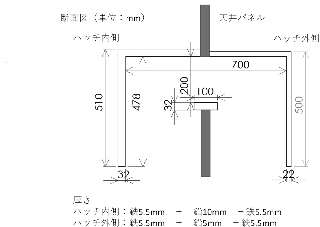
図3 給気ダクト(参考図)
