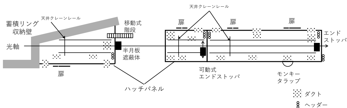
図2 ハッチ構造体の形状(参考図)
