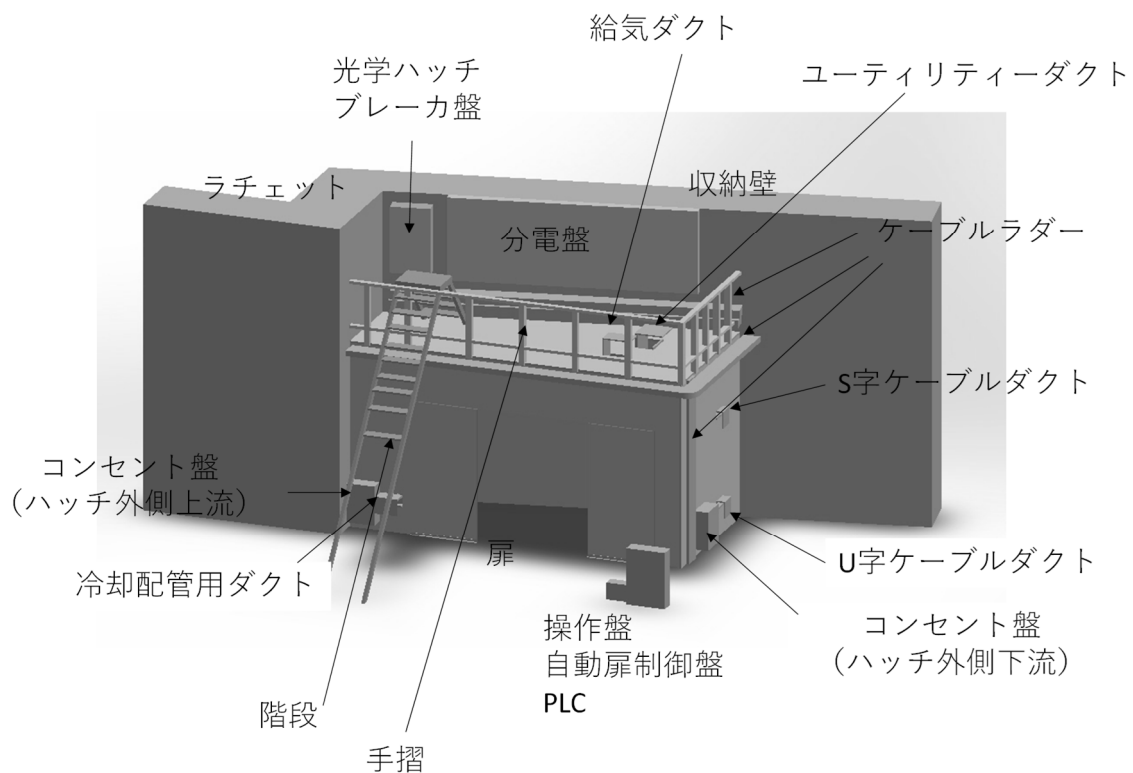
図 1 ハッチの構成要素（参考図）
