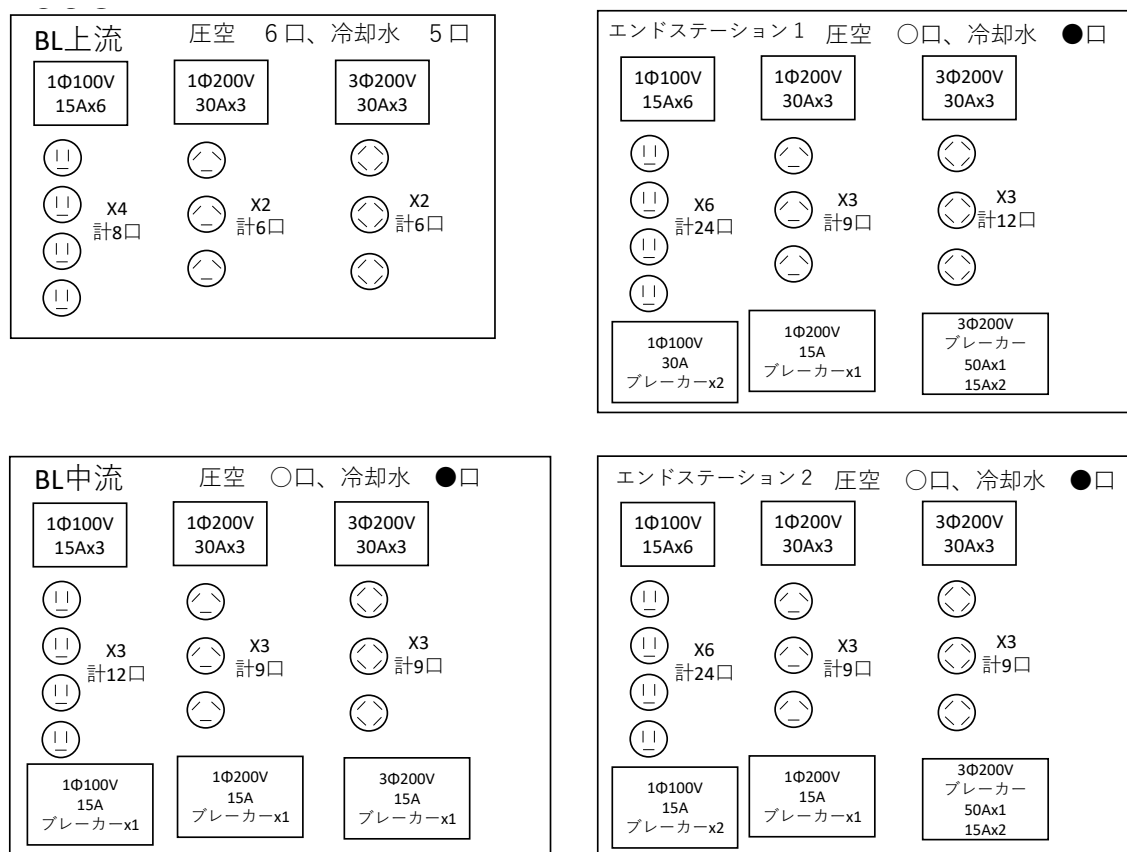
図8 ブレーカ盤の形式
