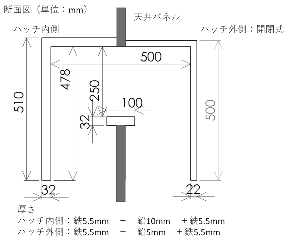
図4 ユーティリティーダクト(参考図)
