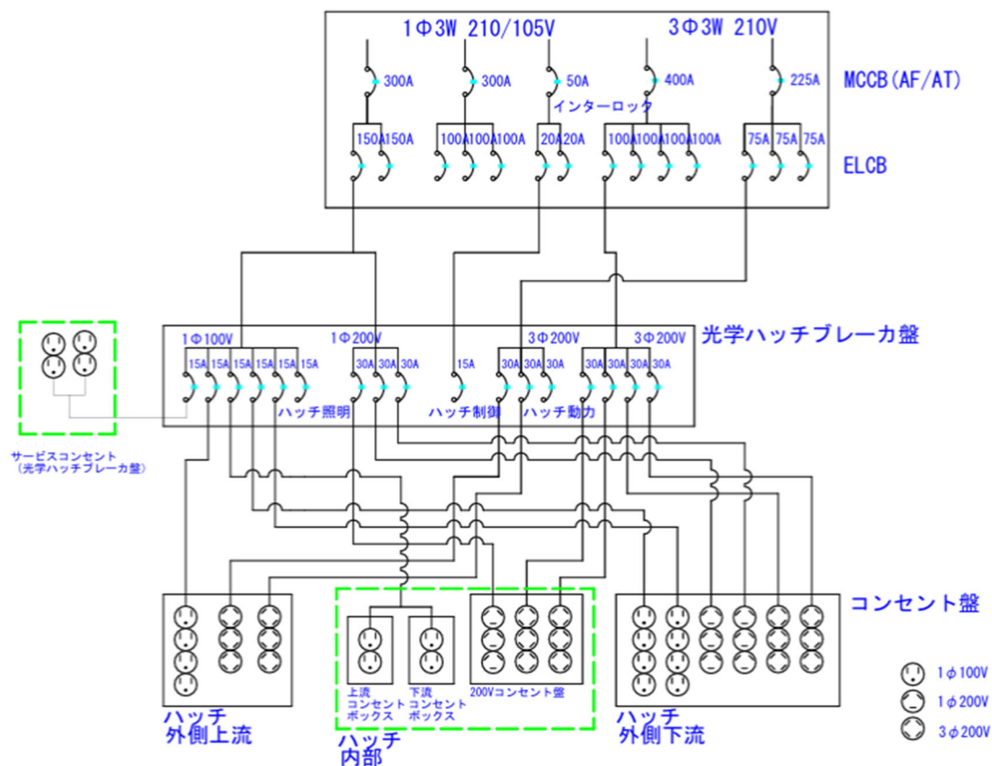
図9 分電盤の取り付け図
