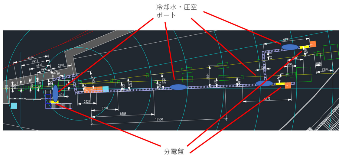
図10 分電盤の配置図
