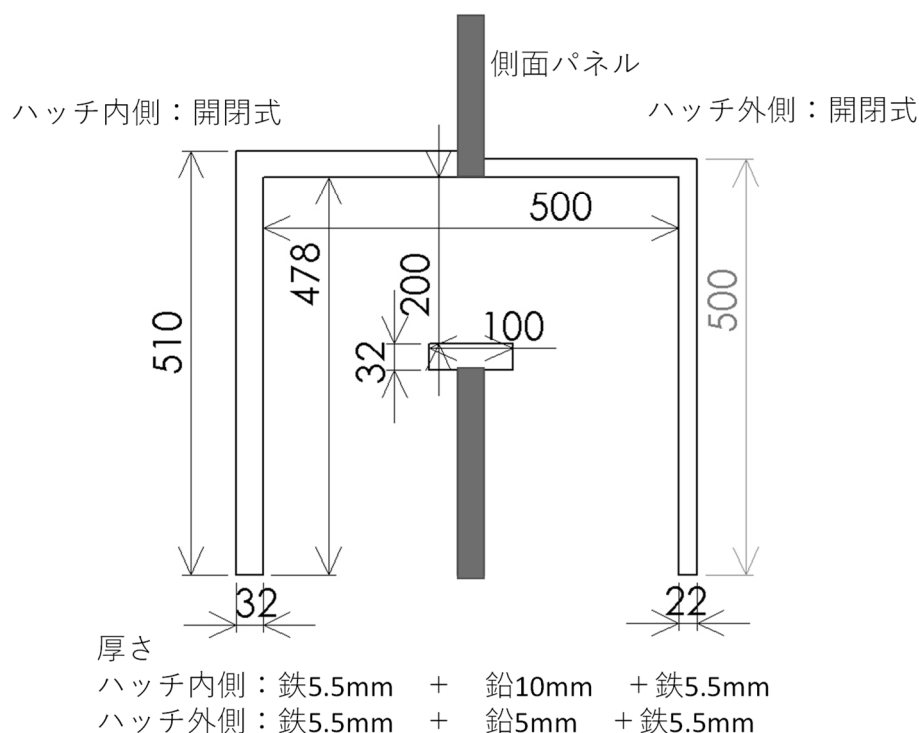
断面図（単位：mm）
