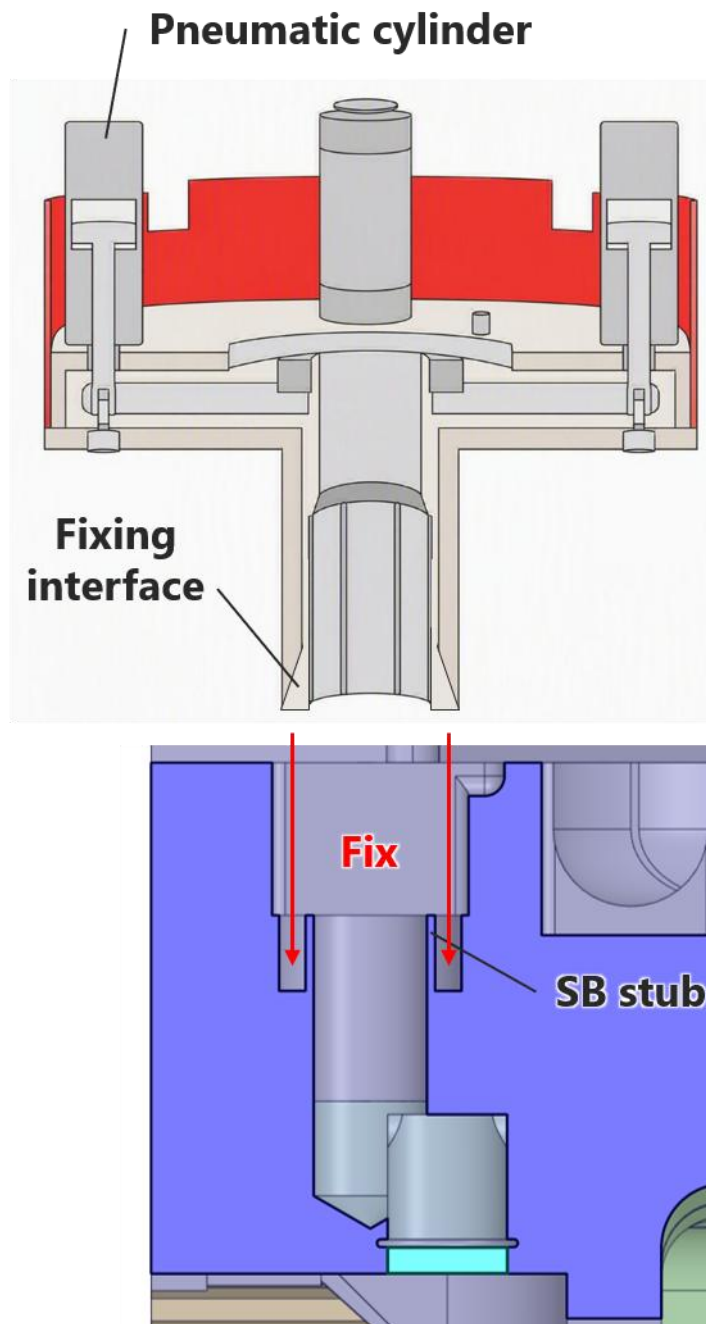
図 23 TPTJ の SB への固定機構部の構造概念図
