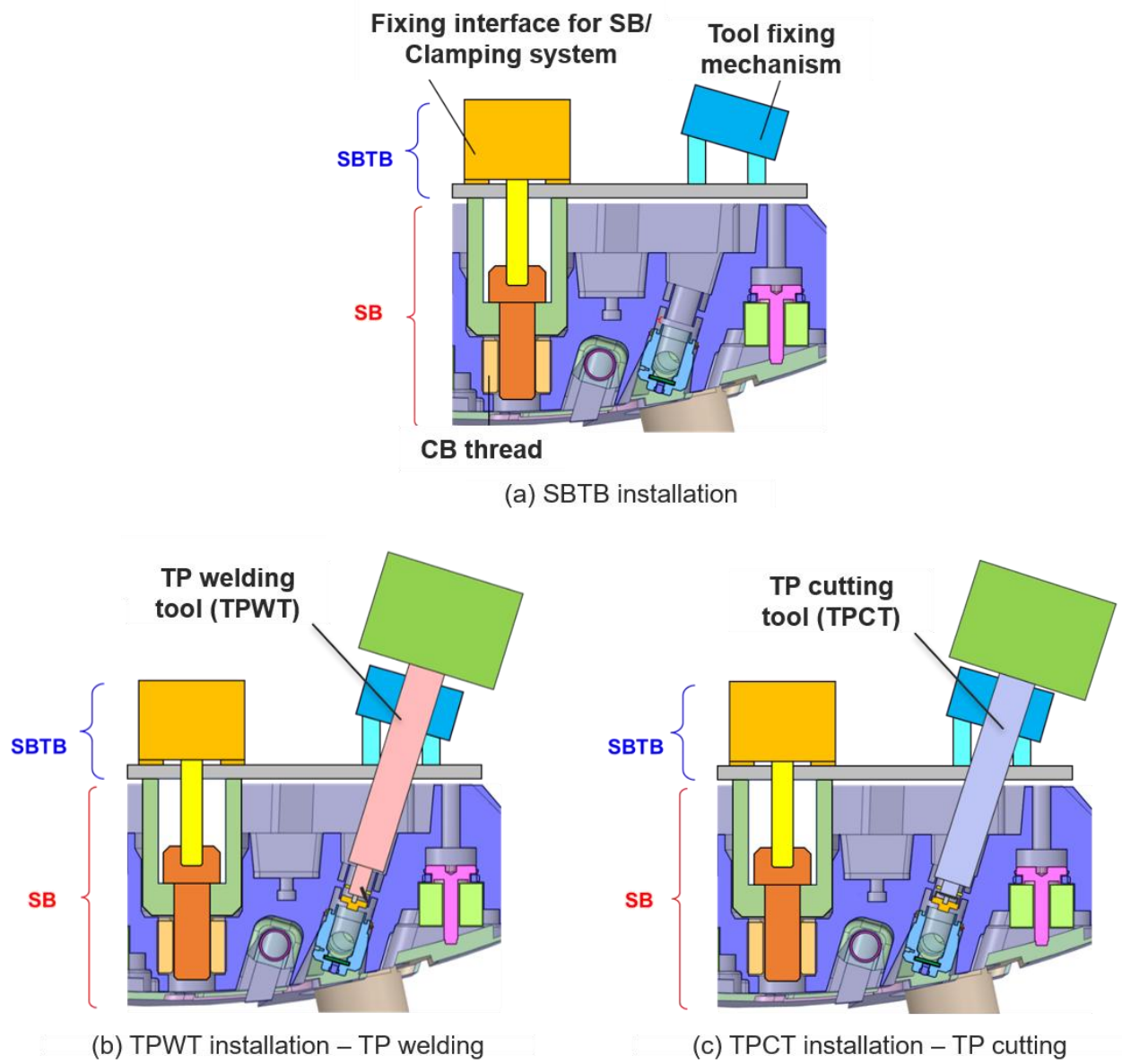
図 8 TP の設置手順その 3
