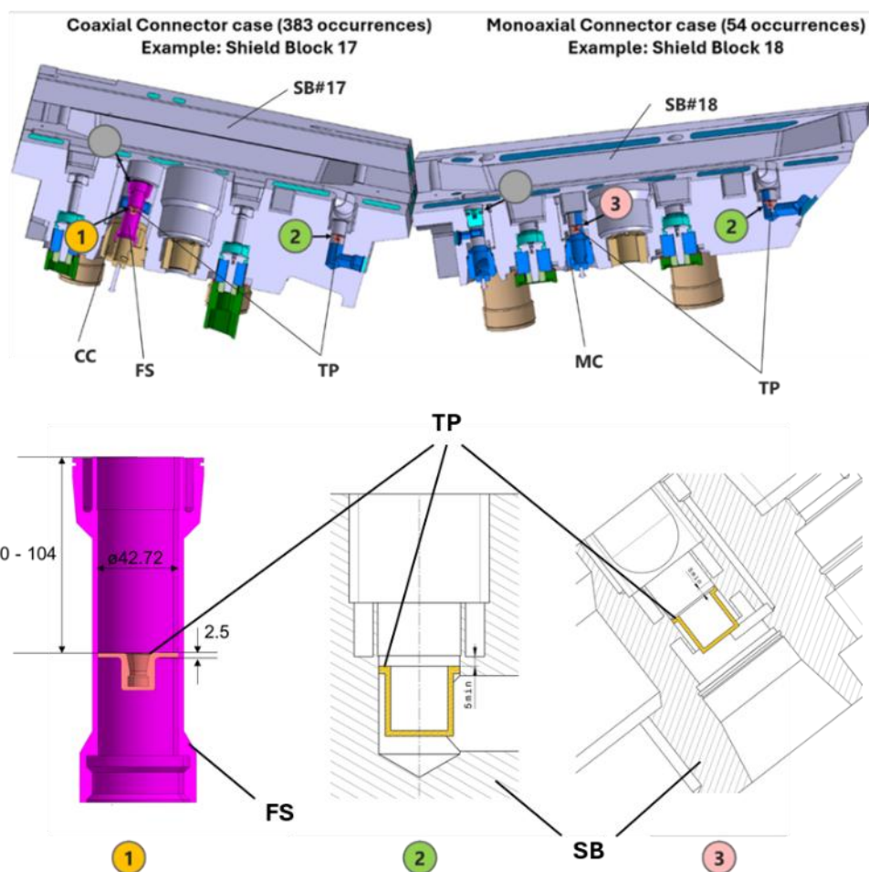
図 5 BM#17 及び #18 におけるプラグ (TP) 設置概略
