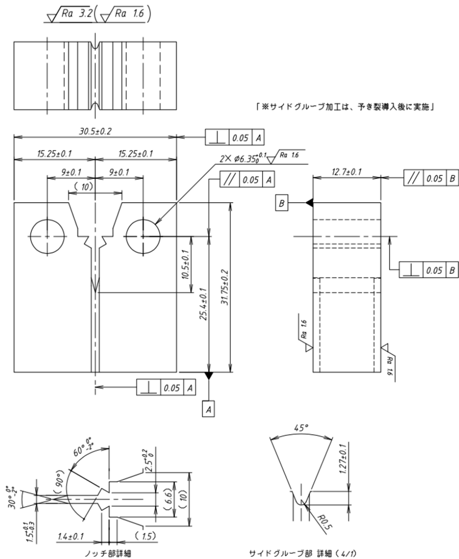
図 2.1 破壊靱性試験片の概略 (例)
