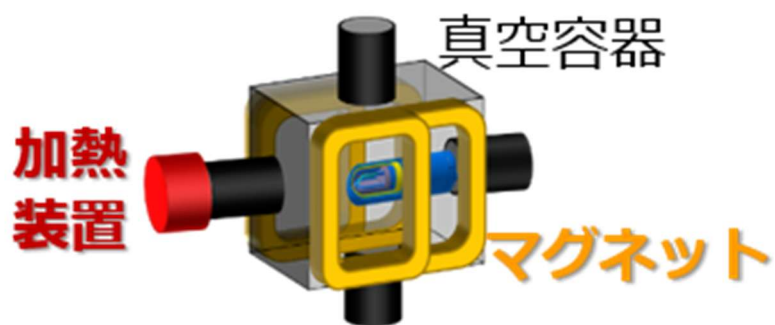
図3 傾斜磁場下熱負荷試験装置の概念図
