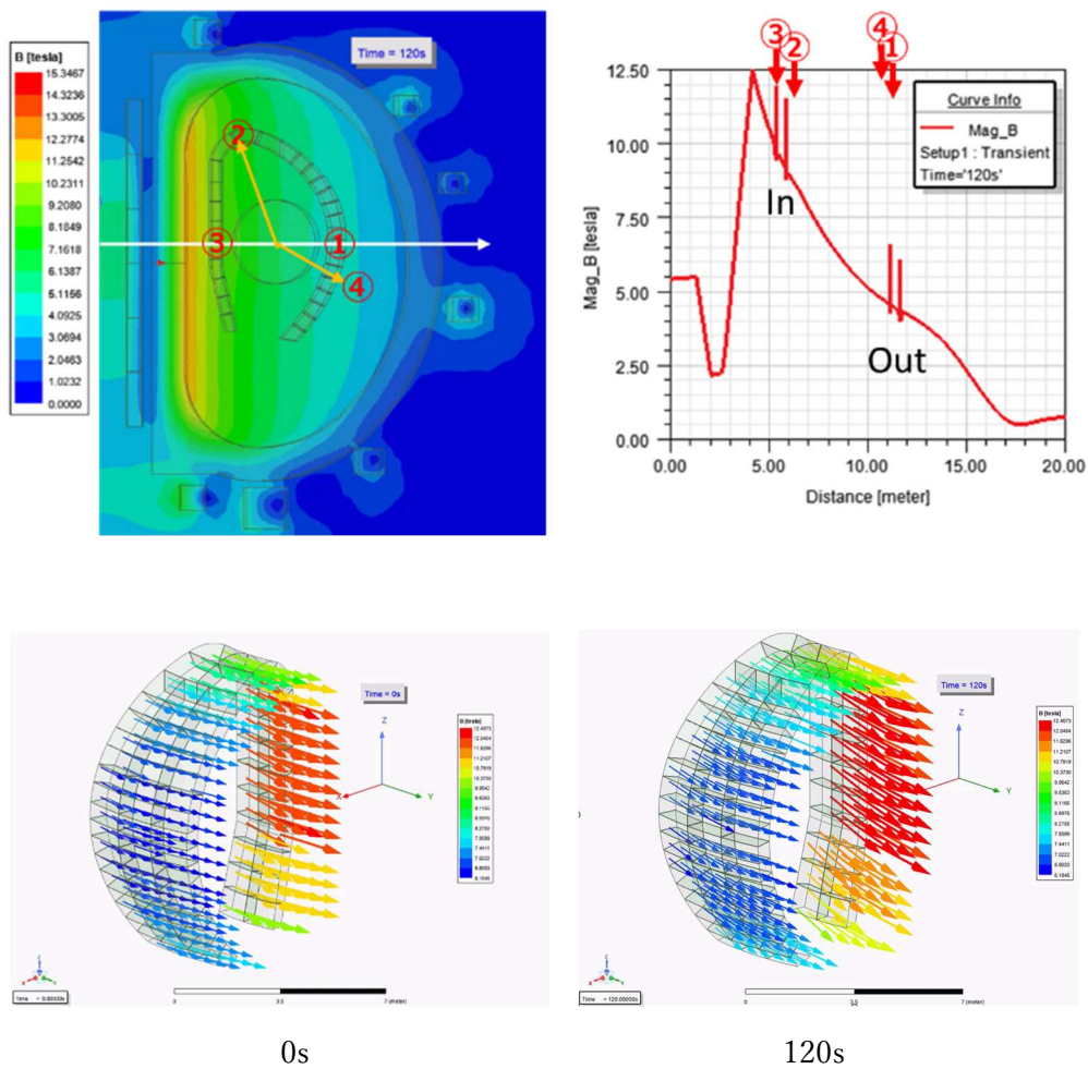
図1 核融合炉内の磁場分布例
