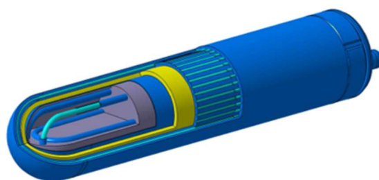
図2 想定するブランケットの概念図 (上) ベリライトブロック設計案 (下) サブモジュール設計案
