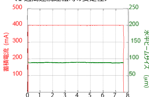
図) 蓄積電流(赤線)と水平電子ビームサイズ(緑線)の時間プロフィール
