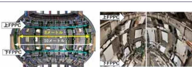
図) JT-60SA 内で完成したFPPC
