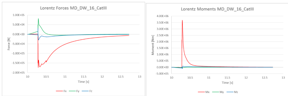
図 3 ディスラプション時に、ある機器に印加するローレンツ力（左）及びモーメント（右）の合計の時間発展
