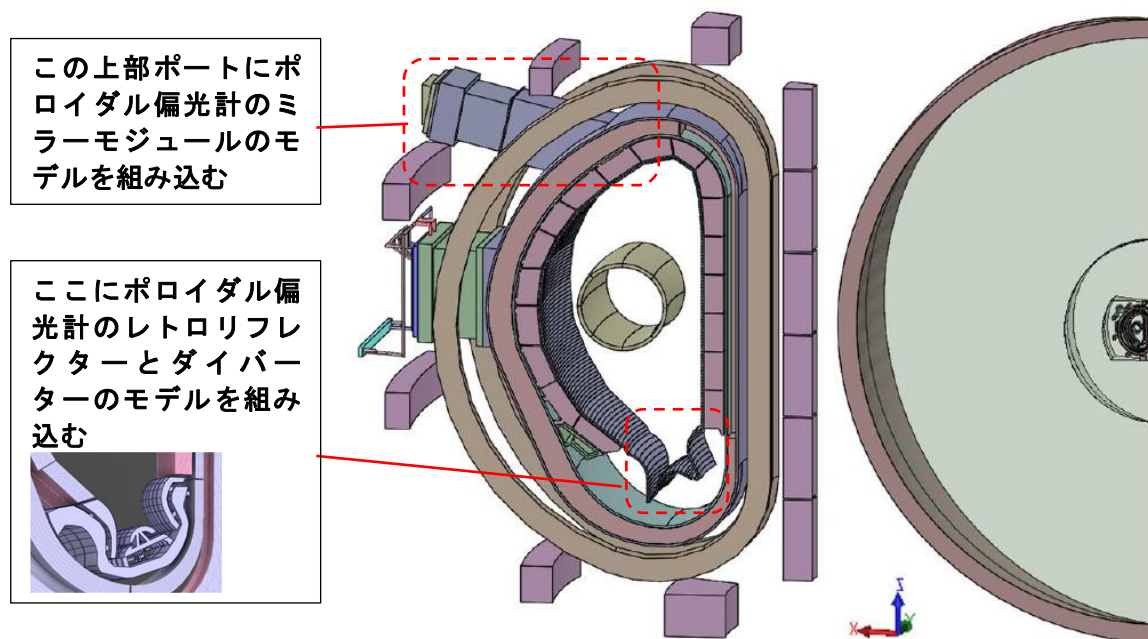
図 1 貸与品の電磁力解析モデル
