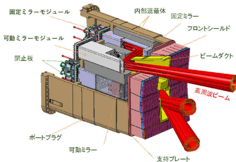
図1 ITER 水平ランチャーの構造
