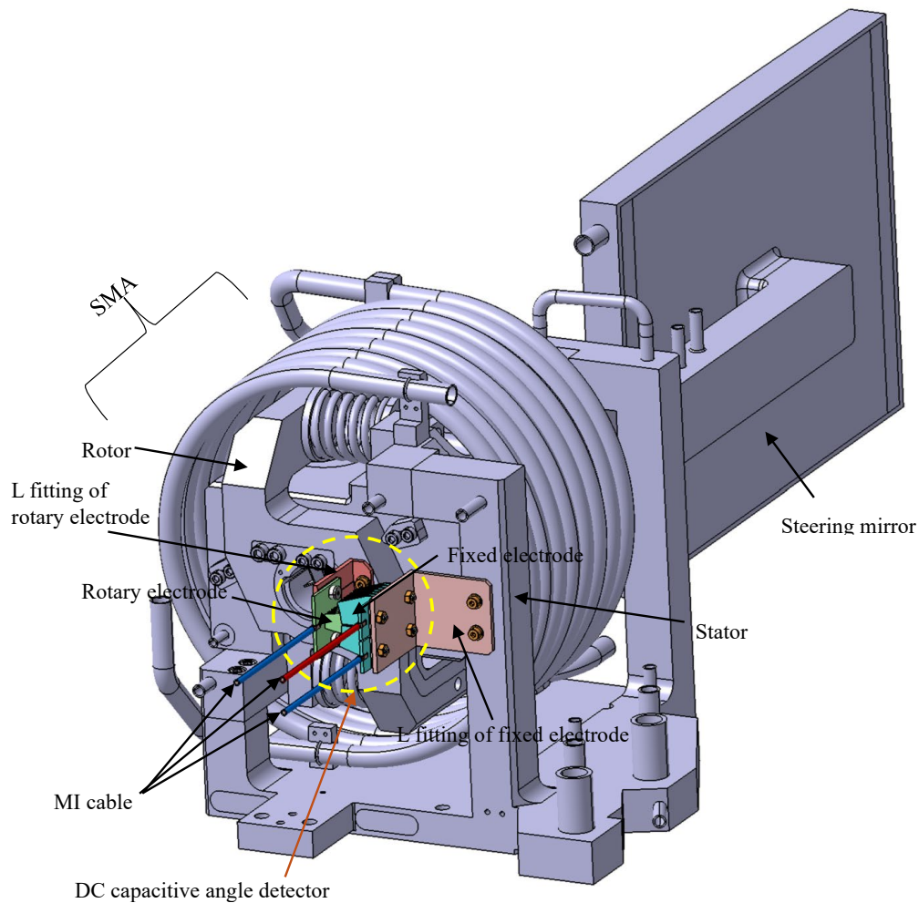
図 2.1-2 SMM における DC 型角度検出器の電極の据付の例
