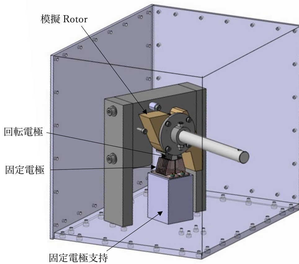
図 2.2-2DC 型角度検出器用電極の Mock-up 装置における据付例
