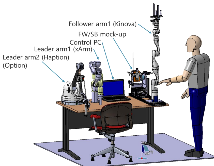
Figure 5 試験構成概念例（フォロワーアームに Kinova を適用した場合）
