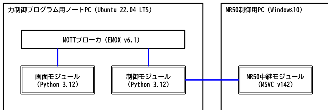
Figure 3 既存制御プログラムソフトウェア構成
