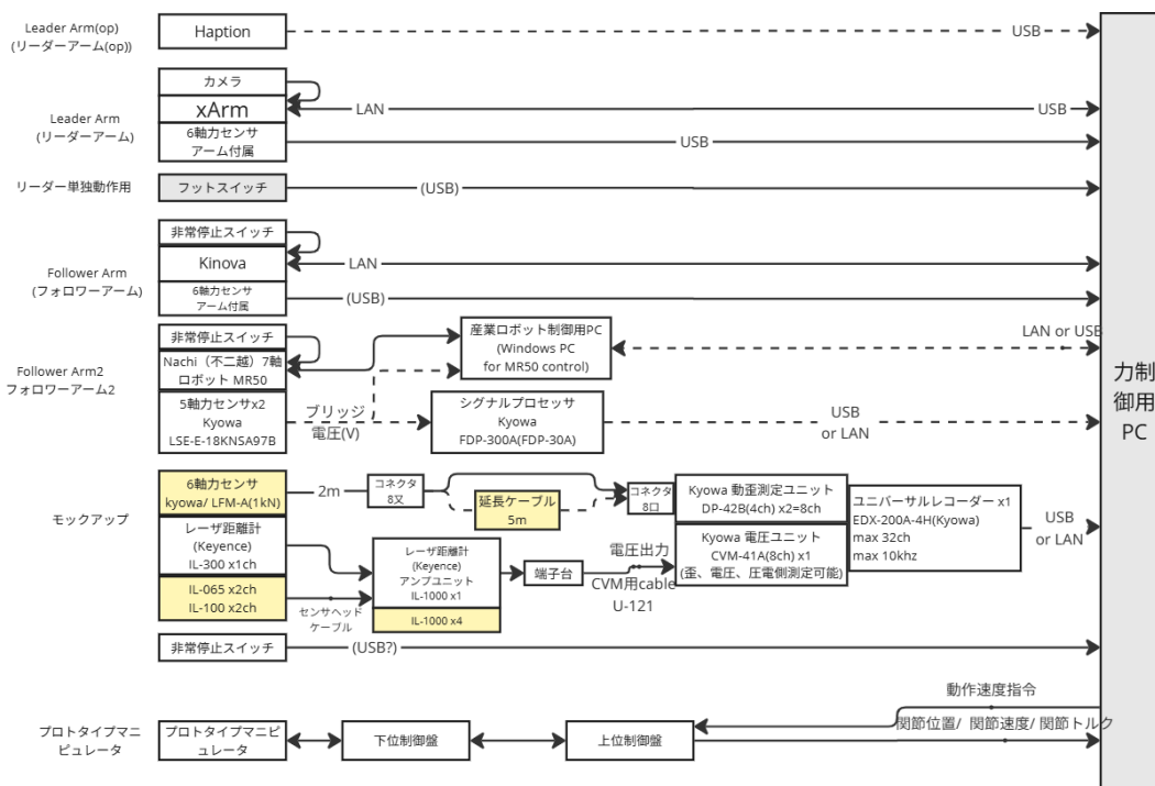
Figure 1 システム構成
