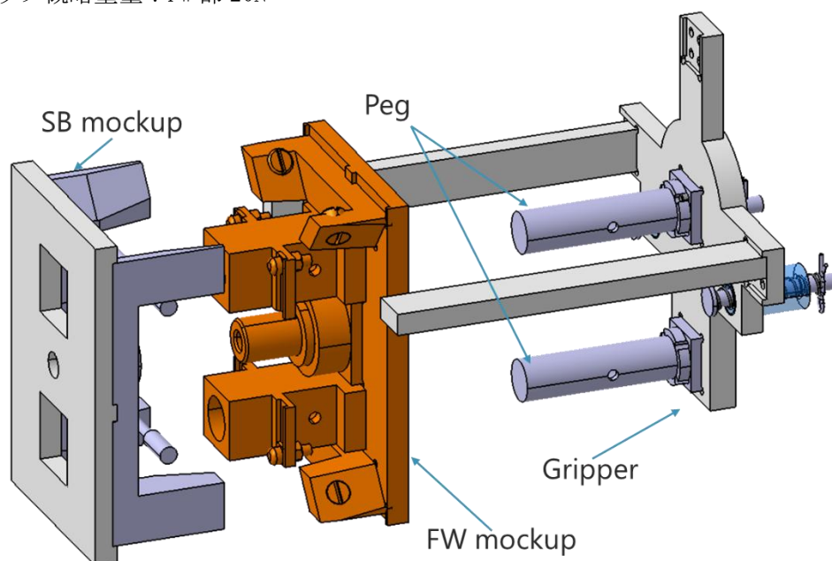
Figure 6 把持爪挿入の試験用モックアップ
