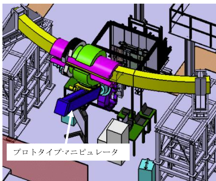
Figure 2 プロトタイプマニピュレータ概念
