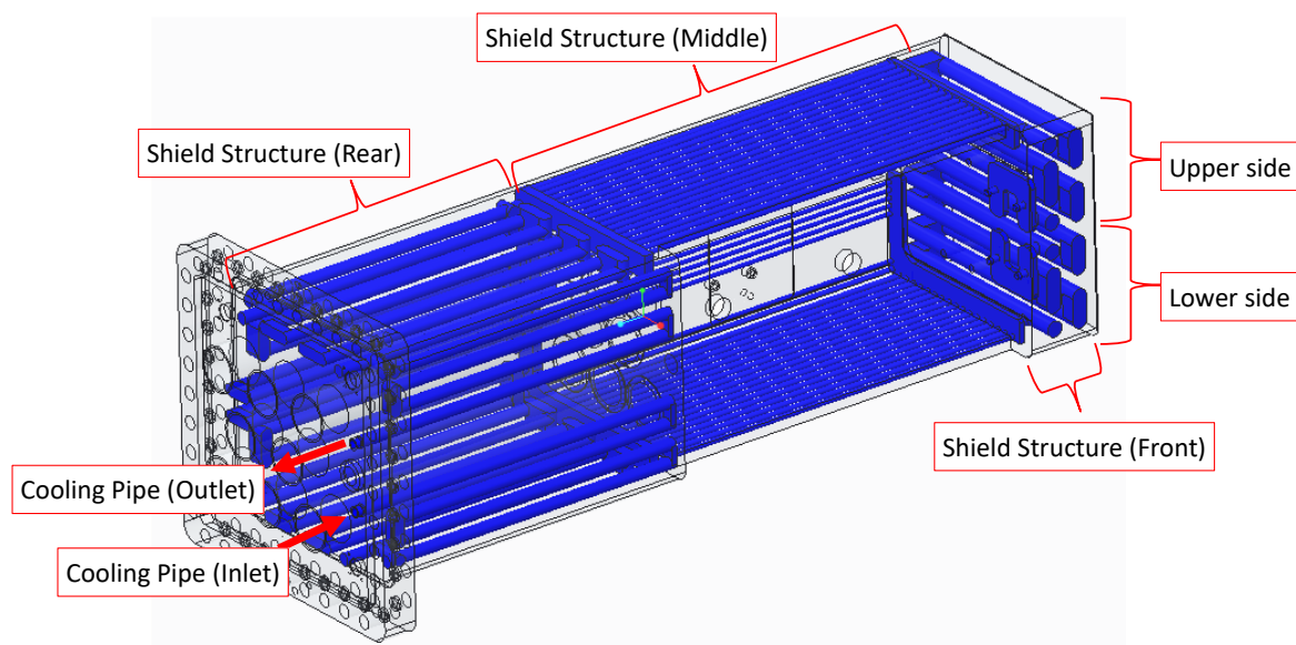
図2 ミラーモジュールの外観及び冷却水流路
