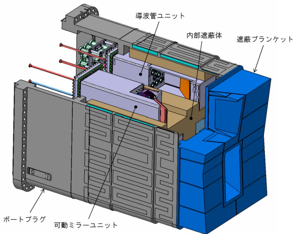
図1 水平ランチャーの構造
