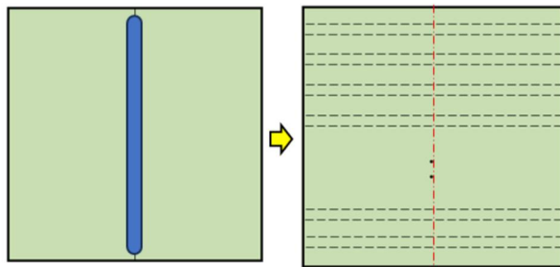
図 3: EBW 溶接部を横断する深穴加工の実施想定図。青色箇所は EBW のビードを示す。
