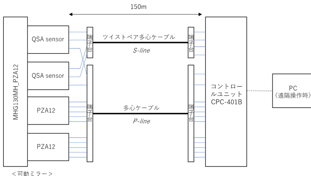
図 1 現状の可動ミラー及びコントローラ類の機器構成
