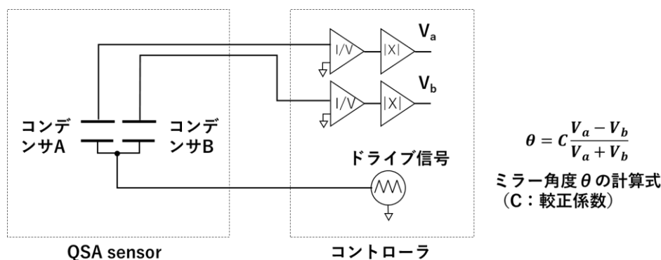
図 3 角度センサの電気回路（模式図）
