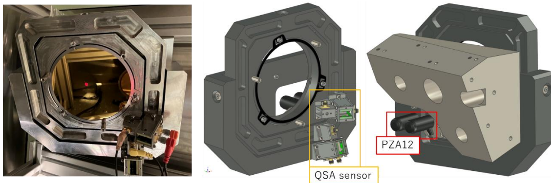
図 2 現状の可動ミラーの外観
