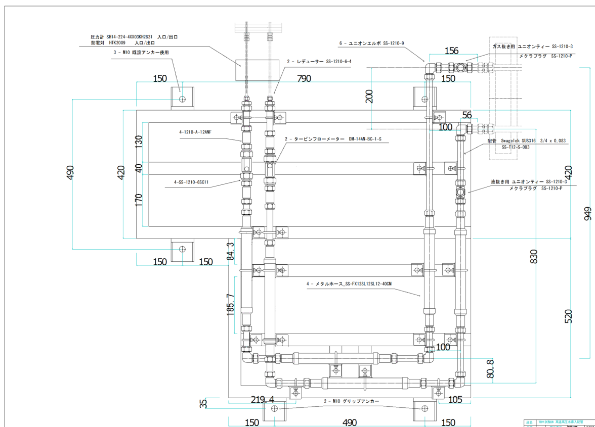
図2 高温高压水導入配管接続部の設計図
