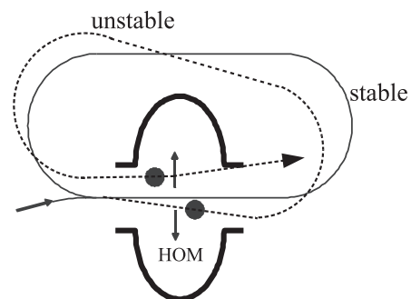
図7 HOM-BBUの原理：先行するバンチが励起した高次モード(HOM)によって後続のバンチが横方向へキックされる。キックされたバンチが周回後にHOMを強める位置と位相で戻ってくると、HOMが指数的に成長し、ビームが失われる。図は単一空洞に簡略化しているが、実際のERLでは多数の空洞が存在する。
