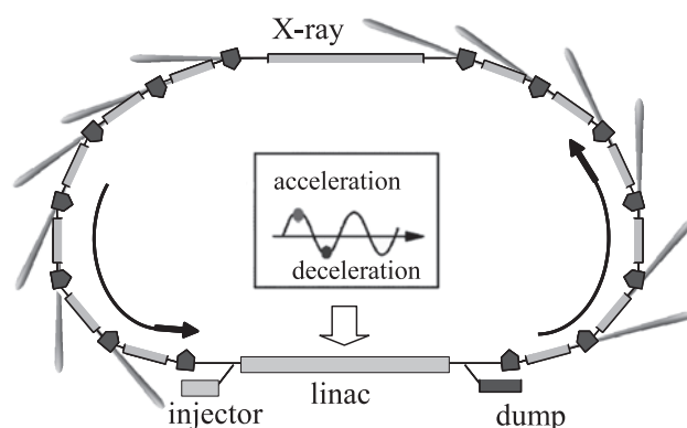
図3 エネルギー回収型リニアックに基づく放射光源の原理. 入射器で発生した電子を超伝導リニアックで加速し, 放射光発生に利用する. 使い終わった電子は, リニアックで減速されビームダンプへ捨てられる. リニアックでは, 加速ビーム, 減速ビームのエネルギー収支がつりあい, 外部からの高周波電力の投入を増やさずに大電流電子ビームの加速が可能になる.
