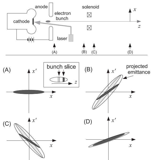
図4 光陰極電子銃を用いたERL入射器における、横方向空間電荷力によるエミッタンス増大とソレノイド磁石によるエミッタンス補償の原理。(A)電子銃直後、(B)電子銃下流＝エミッタンス増大、(C)ソレノイド直後、(D)ソレノイド下流＝エミッタンス補償。
