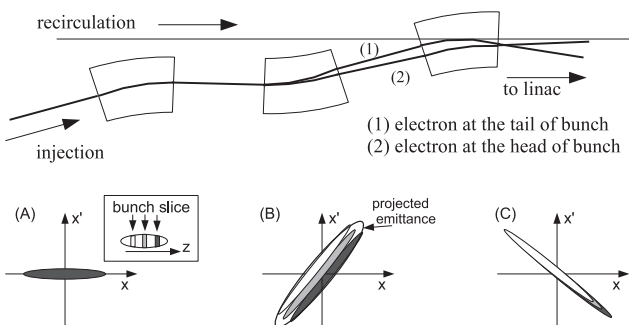
図6 縦方向空間電荷力によるエミッタンス増大とその補償の原理。(A)合流部手前、(B)合流部下流=エミッタンス増大、(C)合流部下流=エンベロープマッチングによるエミッタンス補償を行った場合。合流部の内部で生じる電子バンチのエネルギー再配分により、バンチスライス毎に合流部出口での軌道の不一致が生じる。これによりエミッタンスが増大する。この軌道の不一致を電子ビームのエンベロープと調和させることでエミッタンスの増大を最小にすることができる。この手法をエンベロープマッチングと言う。
