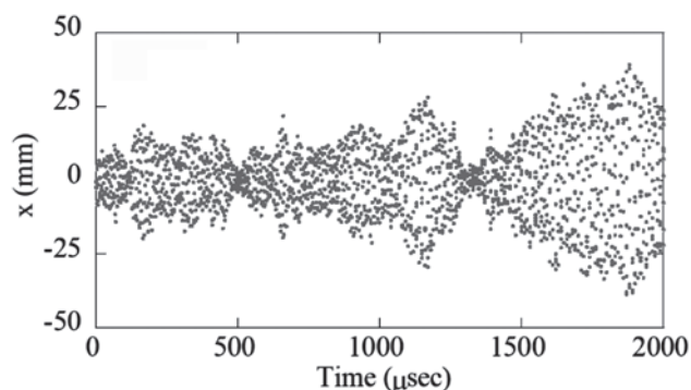
図 8 HOM-BBU の計算例: BBU 閾値を越える電流を加速した場合, 時間とともに電子ビームが横方向に発散する様子が示されている.
