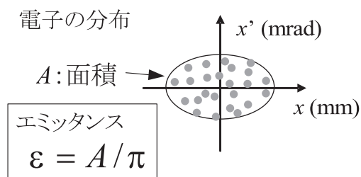
図2 電子ビームエミッタンスの定義. 電子の横方向位相空間(位置と発散角)において, 電子が占める面積を \pi で割った値をエミッタンスと定義する.
