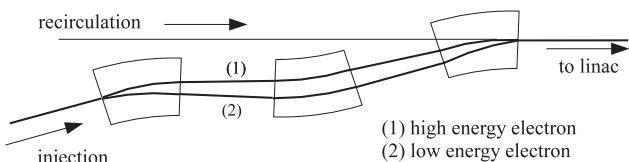
図5 3台の偏向磁石で構成されるERLの合流部。アクロマティックの条件を満たしているため、入射電子にエネルギーの偏差があっても、出射後は同一の軌道になる。
