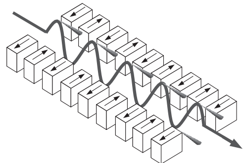
図 1 アンジュレータ放射光の発生。電子ビームは、周期的に交代する磁場中で蛇行運動を行い、蛇行毎に放射光を発生する。その結果、蛇行の周期で決まる振動数にピークを持つ狭帯域の X 線が得られる。
