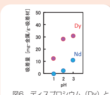
図6 ディスプロシウム(Dy)とネオジウム(Nd)に対する吸着選択性
