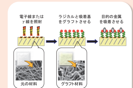
図4 電子線グラフト重合技術
