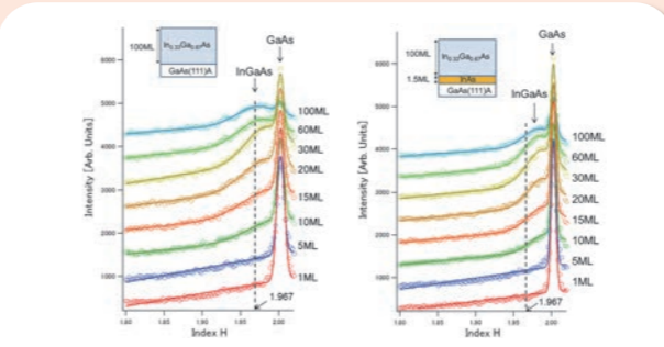
図8 化合物材料の結晶成長プロセスのリアルタイム解析結果(左図:中間層なし、右図:中間層あり)
