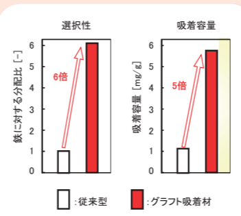
図5 スカンジウムに対する吸着特性
