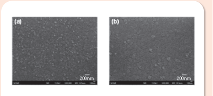
図9 開発したInGaAsの表面写真((a)中間層なし、(b)中間層あり)
