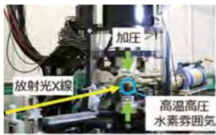
図3 放射光を用いた高温高圧水素雰囲気下の観測装置
