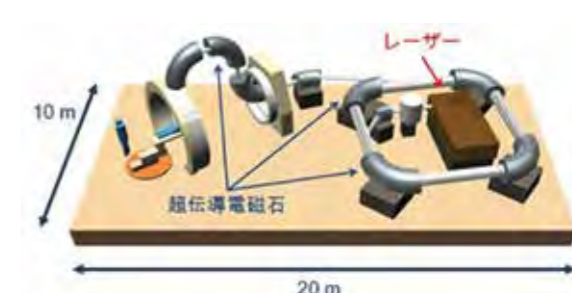
図 4 「量子メス」研究開発により期待される第五世代重粒子線がん治療装置。
