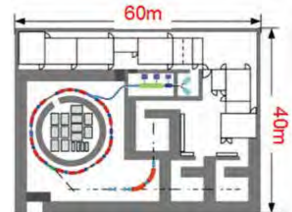
図 3 放医研による普及型小型機の設計。この設計をベースとして 2010 年以降に国内に 3 基が建設され、稼働中。
