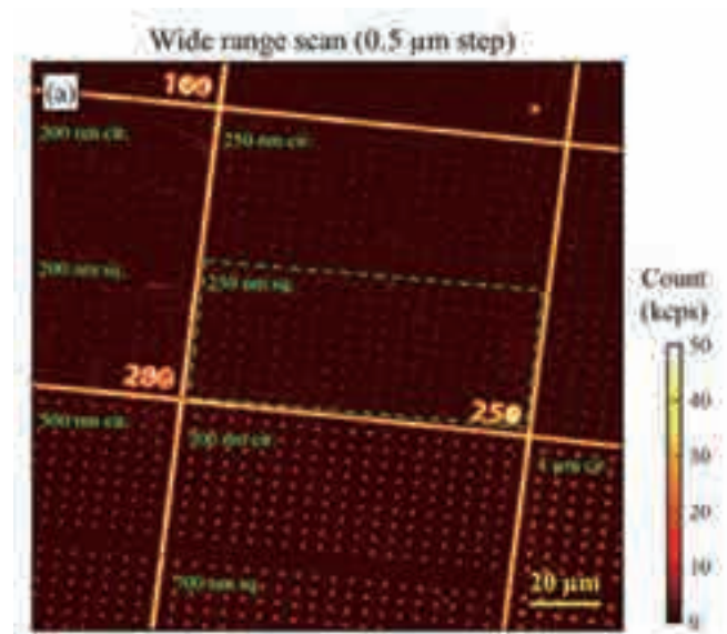
ナノスケール領域に等間隔で注入したNdからの発光マッピング
