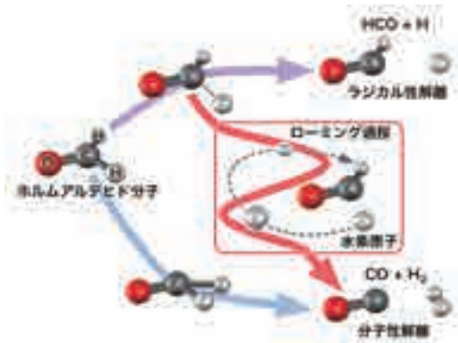
ホルムアルデヒド分子の解離反応の模式図
