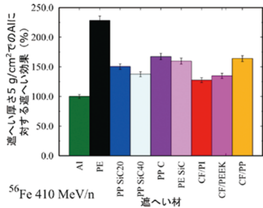
鉄の粒子線を厚さ5 g/cm 2 の材料試料で遮へいしたときの遮へい効果
