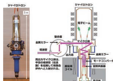
ジャイロトロンの外観及び ジャイロトロンシステムの概要
