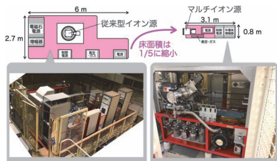
従来型イオン源(左)とマルチイオン源(右)の平面図と写真
