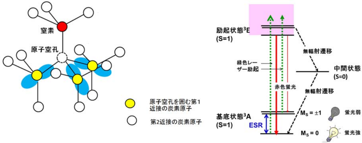
図1: ダイヤモンド中の NV センターの構造とエネルギー準位
